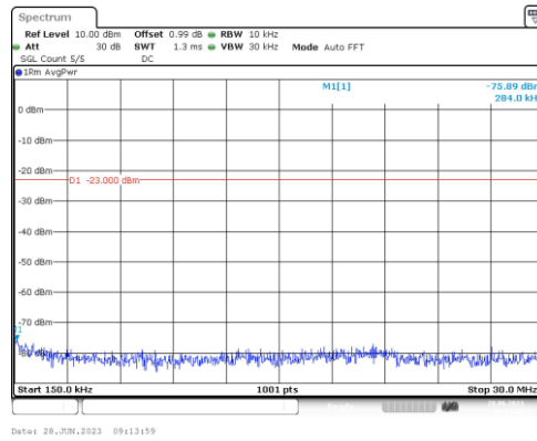
Band71-20MHz-QPSK-133222-1RB#0-Range2:0.15~30MHz
