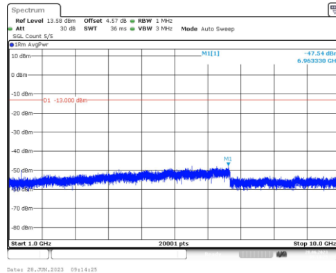
Band71-20MHz-QPSK-133222-1RB#0-Range4:1000~10000MHz
