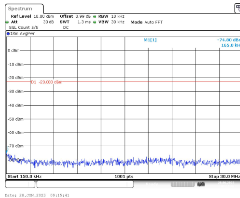
Band71-20MHz-QPSK-133322-1RB#0-Range2:0.15~30MHz
