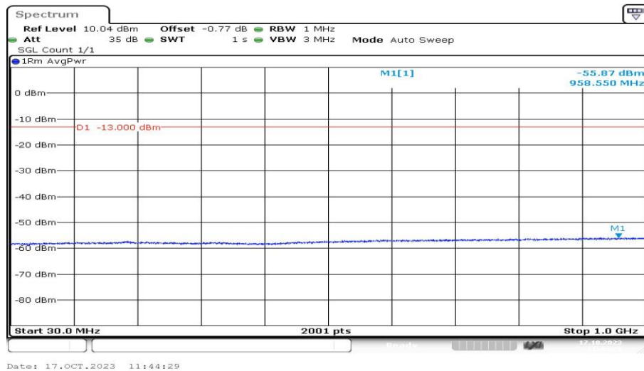
Band4-1513-3-30~1000MHz-PASS
