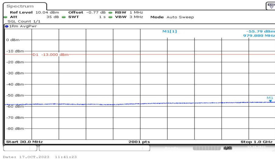
Band4-1513-2-30~1000MHz-PASS
