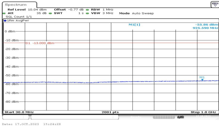
Band4-1413-3-30~1000MHz-PASS
