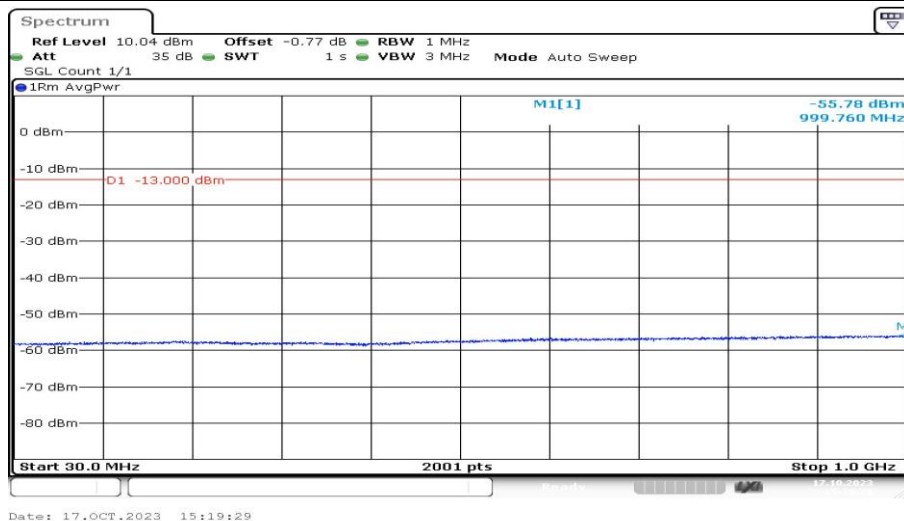
Band4-1413-2-30~1000MHz-PASS
