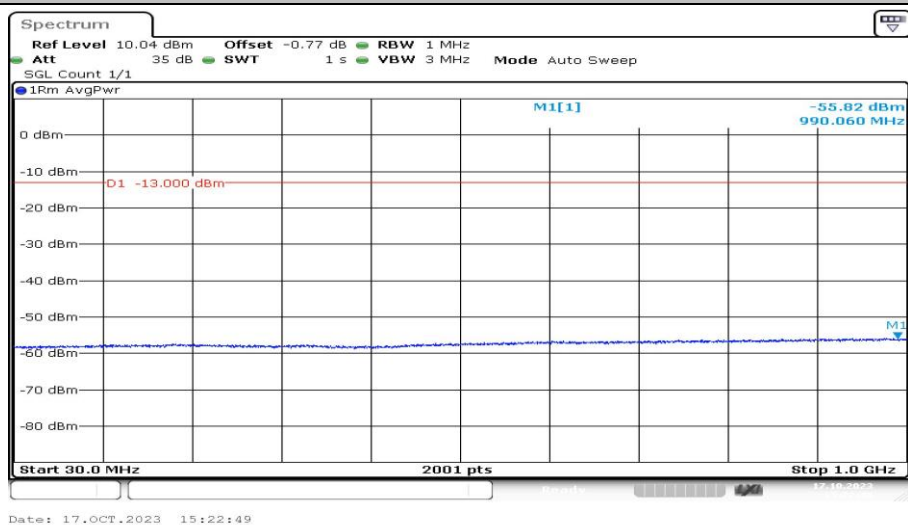
Band4-1312-3-30~1000MHz-PASS
