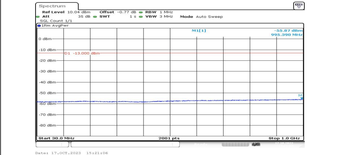
Band4-1513-2-30~1000MHz-PASS
