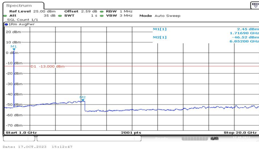
Band4-1312-1-1000~20000MHz-PASS
