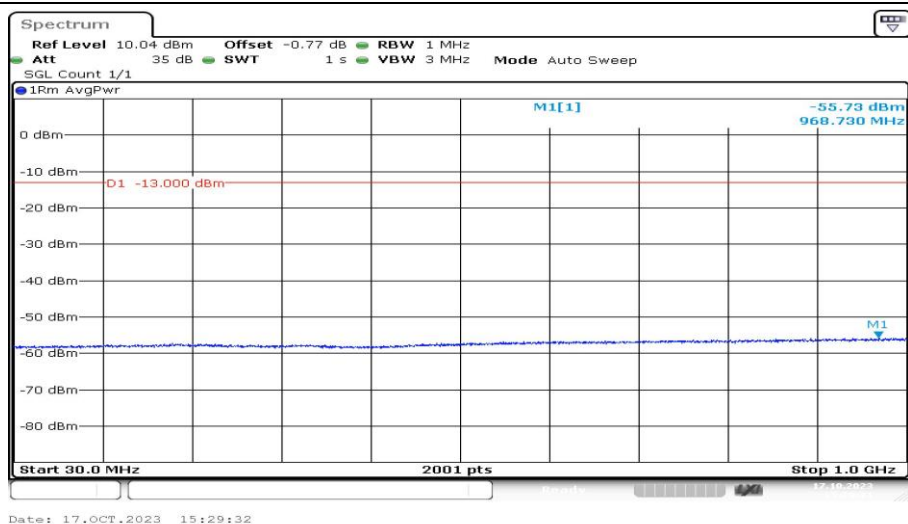
Band4-1413-4-30~1000MHz-PASS
