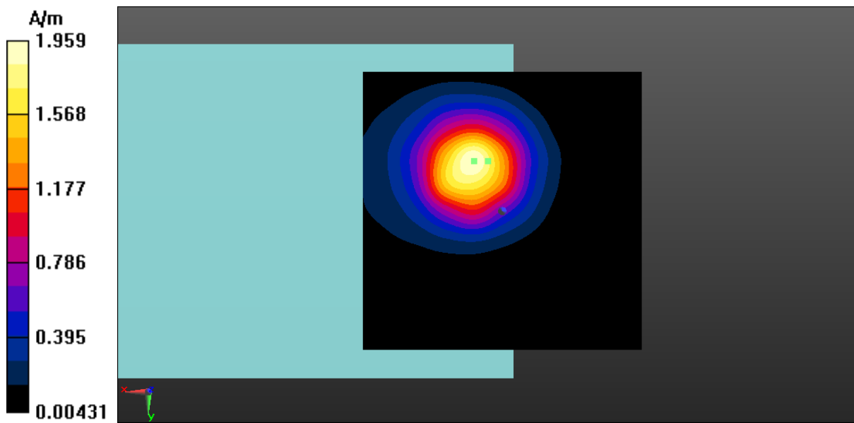
Fig A.20 T-Coil EDGE 850-Z
