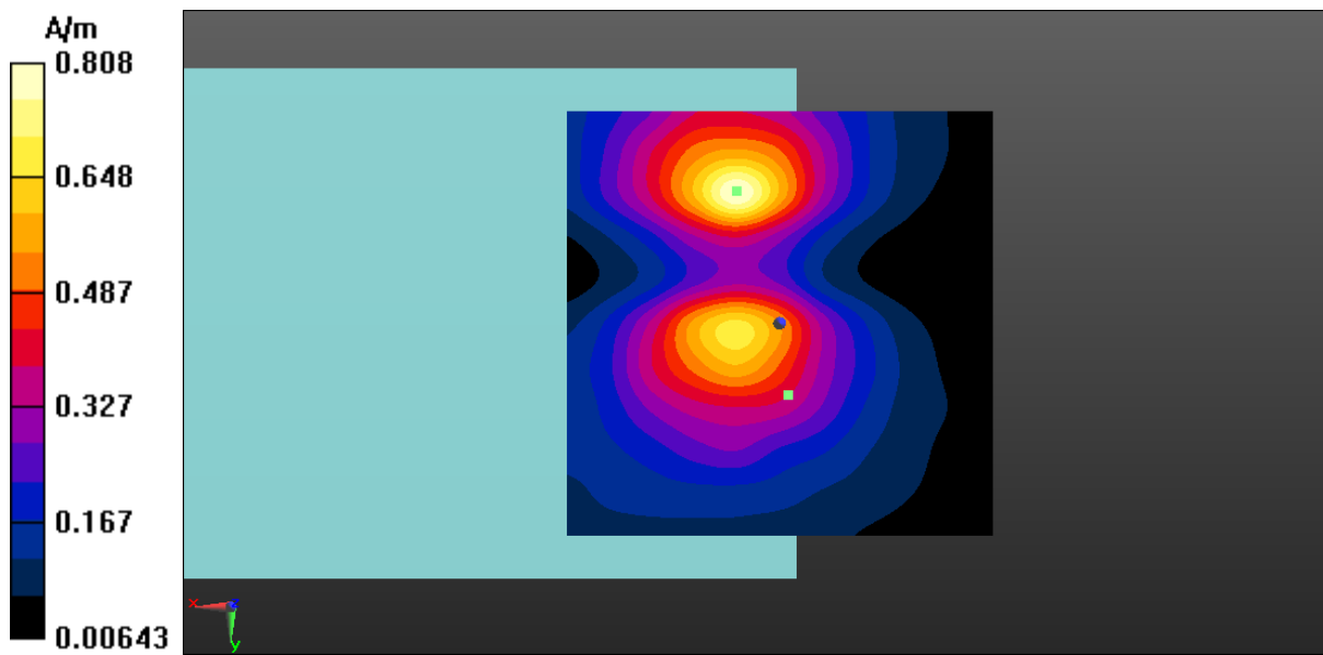
Fig A.20 T-Coil EDGE 850-Y
