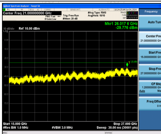
Band41-5MHz-QPSK-41565-1RB#0-Range3:15000~27000MHz
