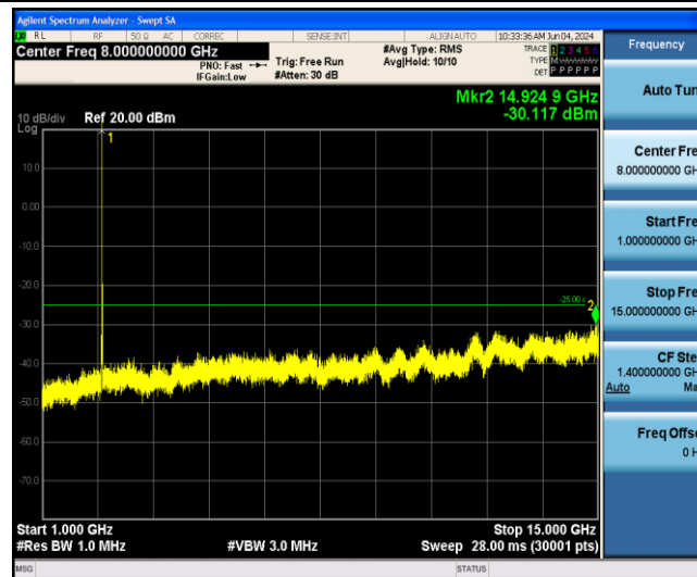
Band41-10MHz-QPSK-39700-1RB#0-Range2:1000~15000MHz
