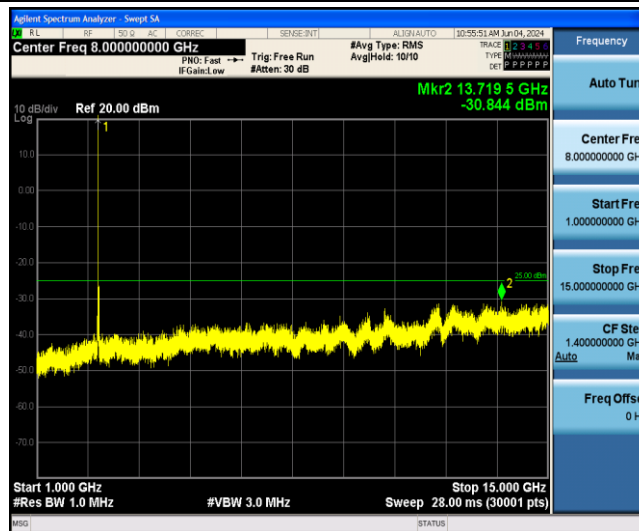
Band41-20MHz-QPSK-41490-1RB#0-Range2:1000~15000MHz
