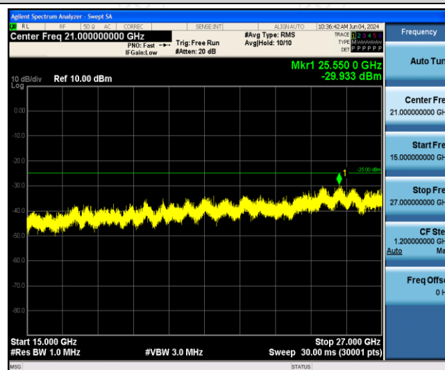
Band41-10MHz-QPSK-41540-1RB#0-Range3:15000~27000MHz
