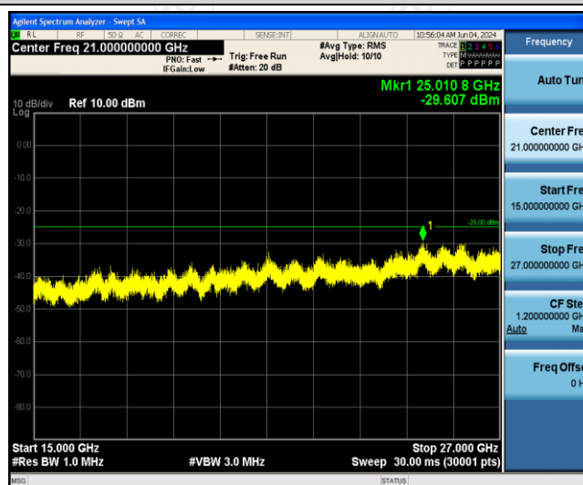
Band41-20MHz-QPSK-41490-1RB#0-Range3:15000~27000MHz
