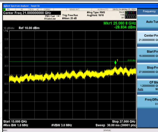
Band41-5MHz-QPSK-41565-1RB#0-Range3:15000~27000MHz
