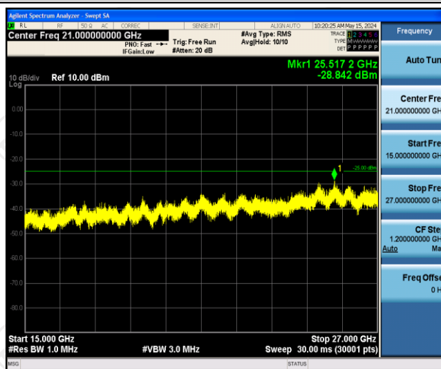
Band41-20MHz-QPSK-41490-1RB#0-Range3:15000~27000MHz
