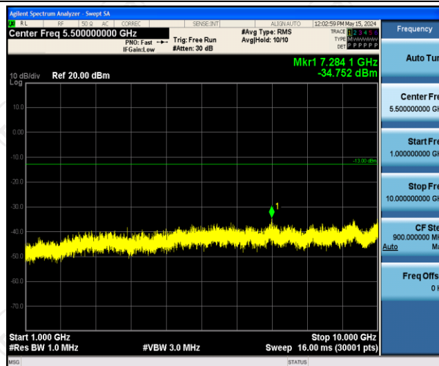
Band71-20MHz-QPSK-133372-1RB#0-Range2:1000~10000MHz
