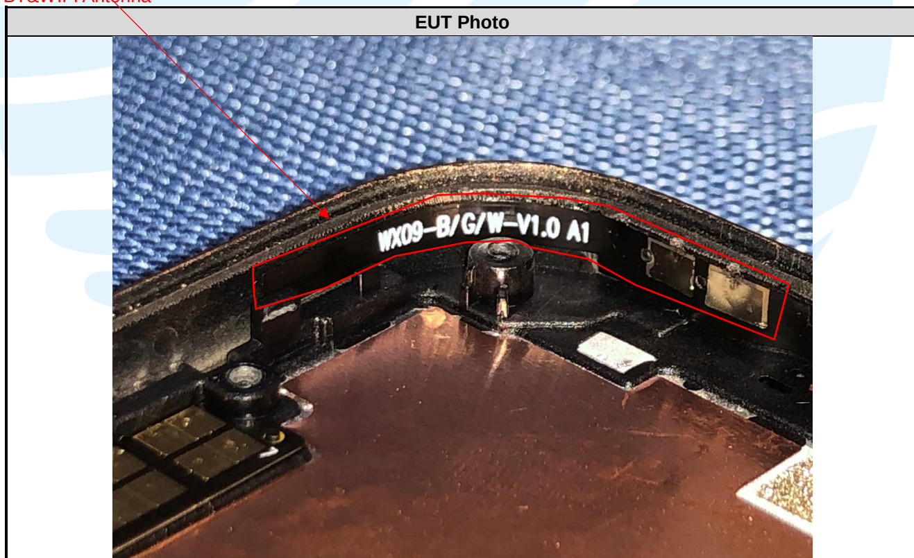
BT&WIFI Antenna
