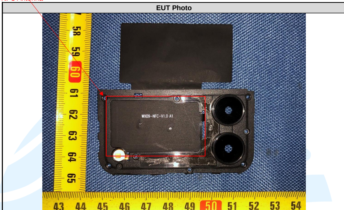
NFC Antenna
