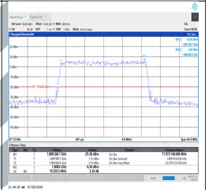
Band2-20MHz-QPSK-19100-100RB#0-PASS
