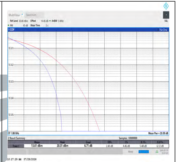
Band2-5MHz-QPSK-18900-25RB#0-PASS
