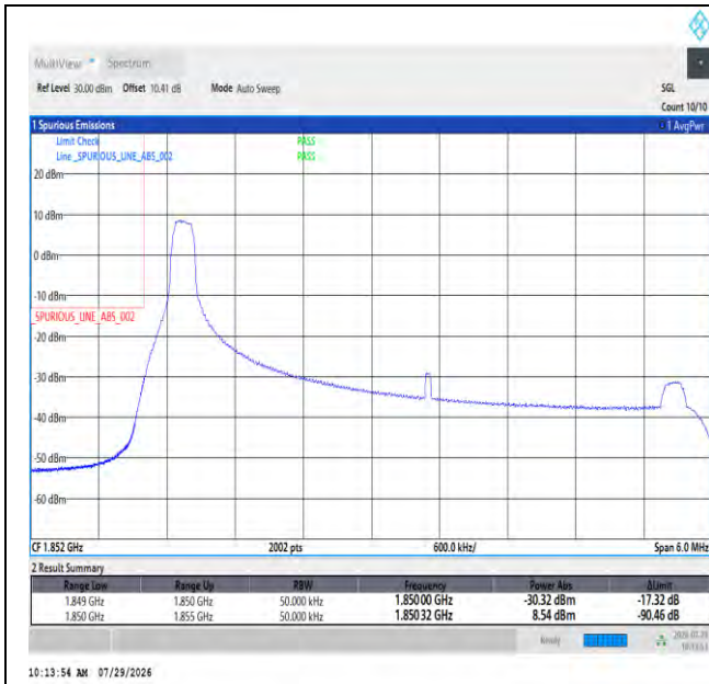
Band2-5MHz-QPSK-18625-1RB#0-PASS
