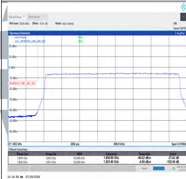
Band2-5MHz-QPSK-18625-25RB#0-PASS
