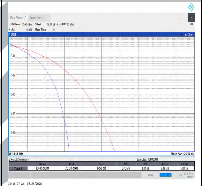
Band2-10MHz-QPSK-18650-50RB#0-PASS
