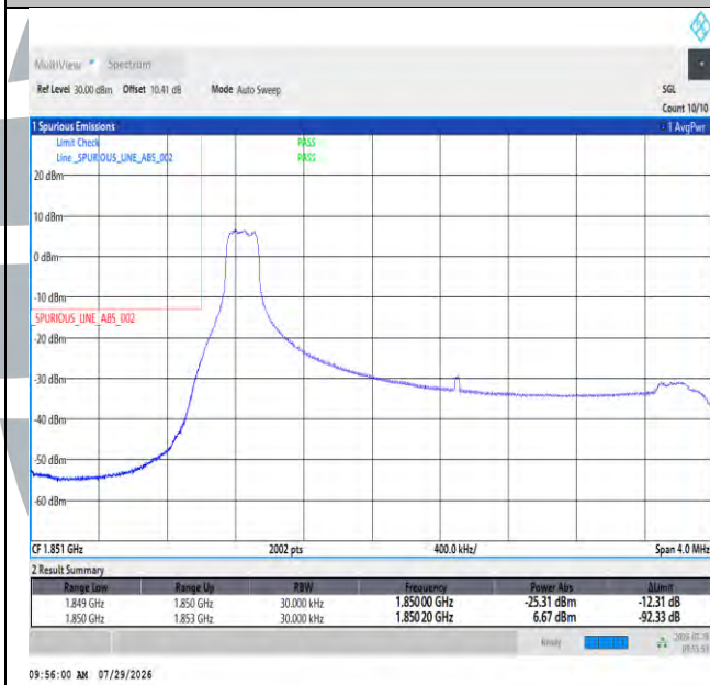
Band2-3MHz-QPSK-18615-1RB#0-PASS
