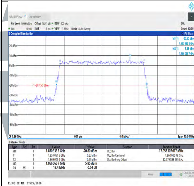
Band2-20MHz-16QAM-18700-100RB#0-PASS
