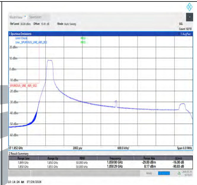
Band2-5MHz-16QAM-18625-1RB#0-PASS
