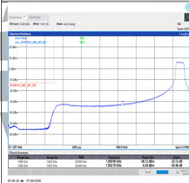
Band2-3MHz-16QAM-18615-1RB#14-PASS
