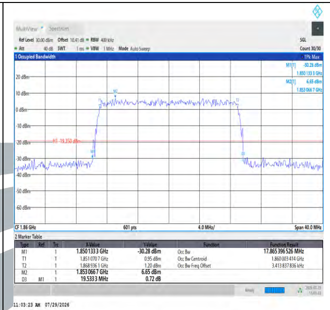
Band2-20MHz-QPSK-18700-100RB#0-PASS
