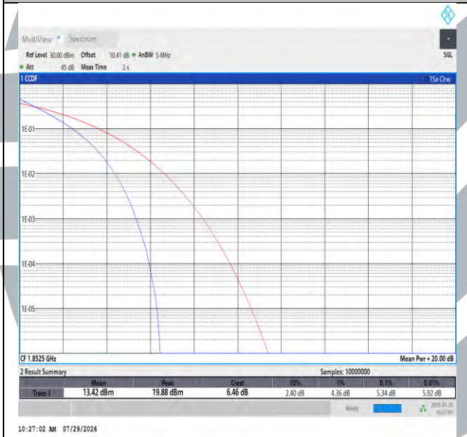
Band2-5MHz-QPSK-18625-25RB#0-PASS
