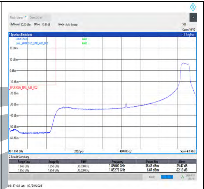
Band2-3MHz-QPSK-18615-1RB#14-PASS
