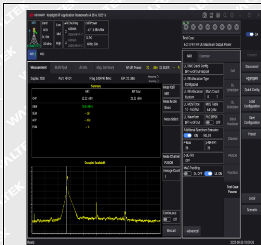
NTNV-N78-3450-3550-PC2-30-20-L-DFT-16QAM- Edge_1RB_Left-PASS
