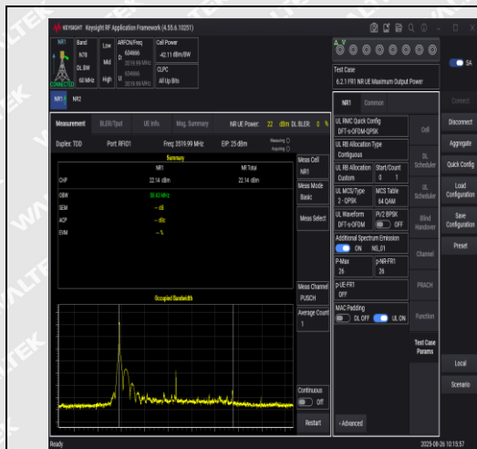
NTNV-N78-3450-3550-PC2-30-60-H-DFT-QPSK- Edge_1RB_Left-PASS
