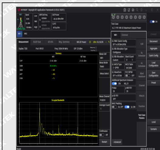
NTNV-N78-3450-3550-PC2-30-90-H-DFT-QPSK- Edge_1RB_Left-PASS
