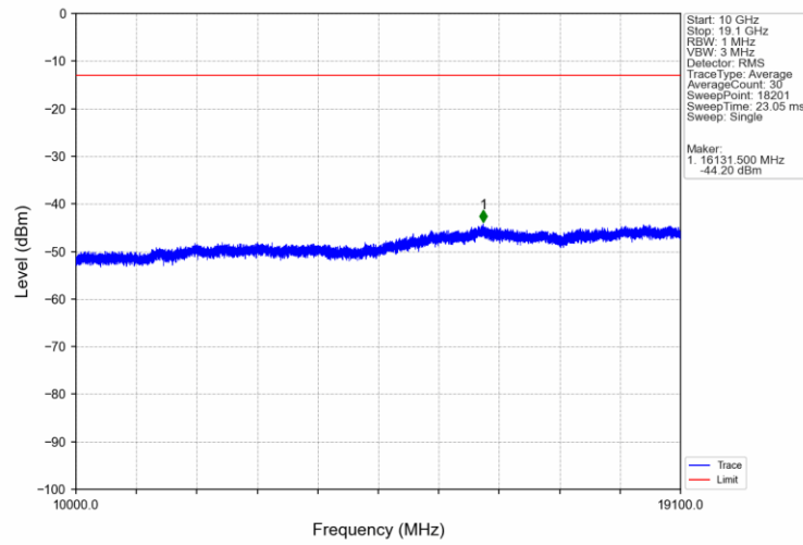
Band2 10MHz 16QAM HCH 1905MHz RB 1 0 NTV
