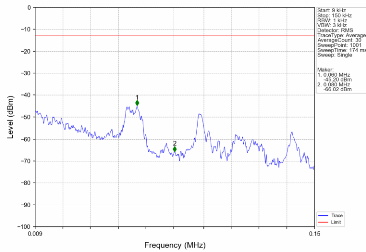
Band2 10MHz 16QAM HCH 1905MHz RB 1 0 NTV
