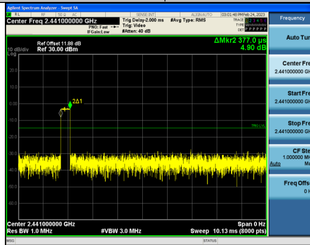
DH3-Ant1-Hop-1.642-160
