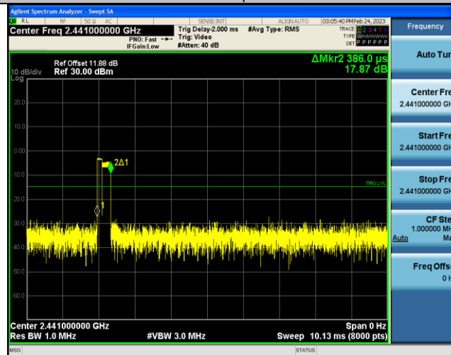
2DH3-Ant1-Hop-1.638-160
