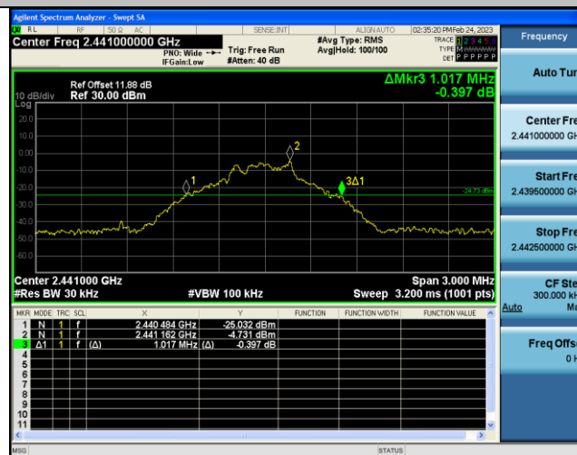
DH5-Ant1-2441
