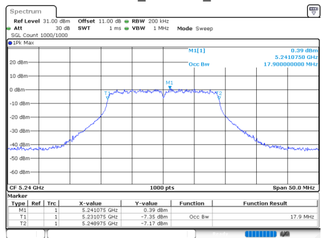
802.11ac20_5240MHz_Chain 0
