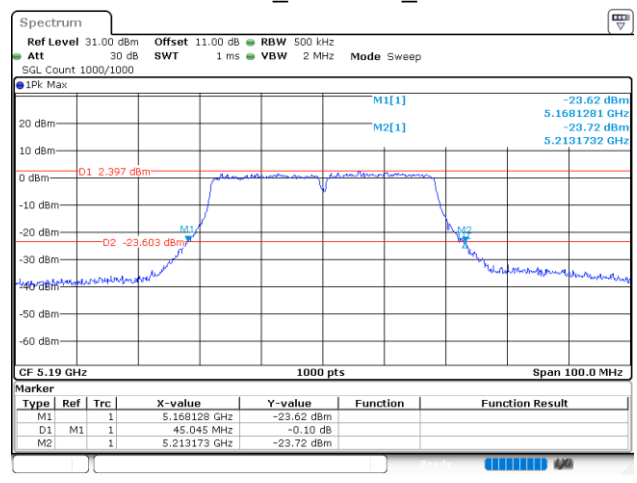
802.11ac40_5190MHz_Chain 1
