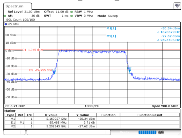
802.11ac80_5210MHz_Chain 0
