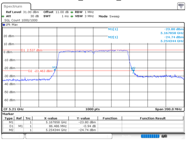
802.11ac80_5210MHz_Chain 1
