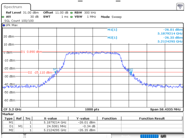
802.11ac20_5200MHz_Chain 0
