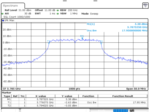
802.11ac20_5785MHz_Chain 0
