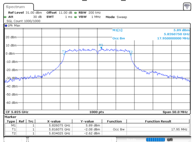
802.11ac20_5825MHz_Chain 0
