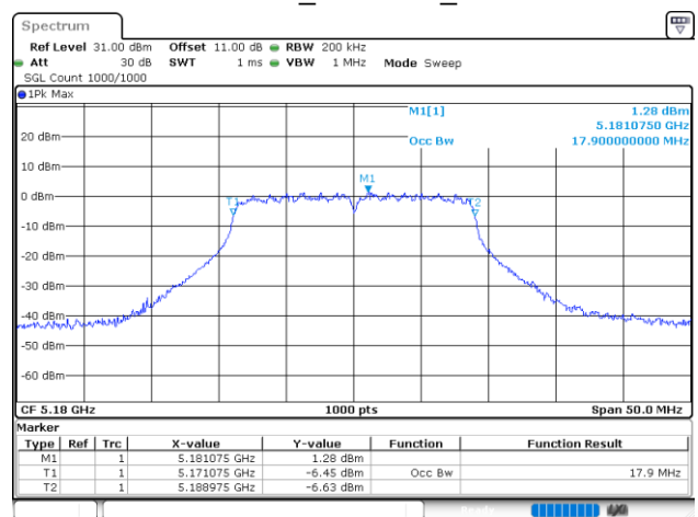
802.11ac20_5180MHz_Chain 0
