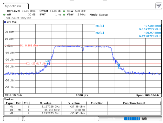
802.11ac40_5190MHz_Chain 0
