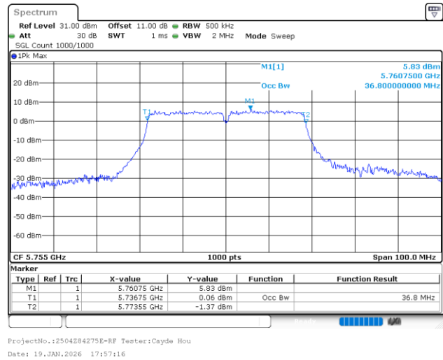
802.11ac40_5755MHz_Chain 1
