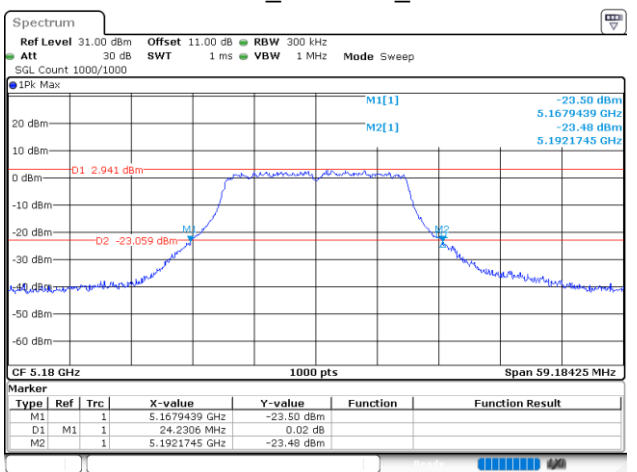
802.11ac20_5180MHz_Chain 1
