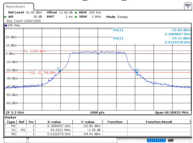
802.11ac20_5200MHz_Chain 1
