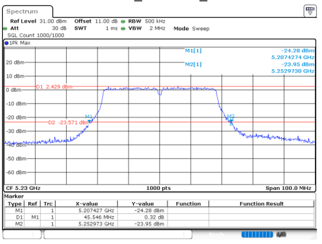
802.11ac40_5230MHz_Chain 1
