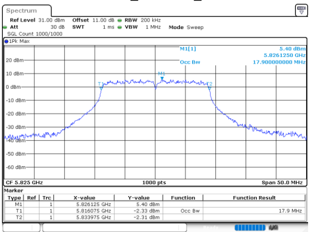
802.11ac20_5825MHz_Chain 1
