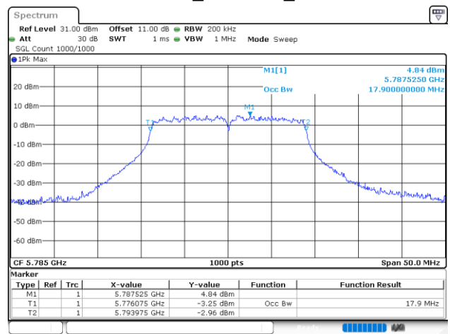
802.11ac20_5785MHz_Chain 1
