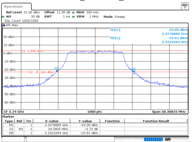
802.11ac20_5240MHz_Chain 1
