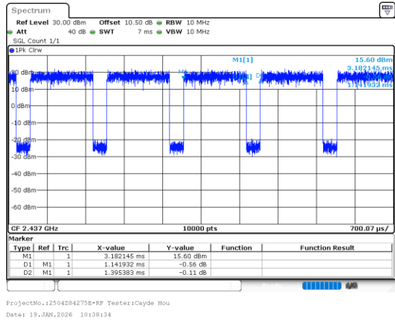
802.11n20_2437MHz_Chain 0
