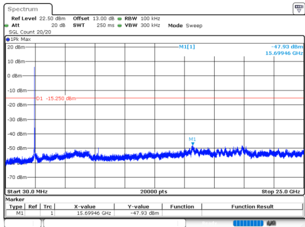
802.11b_2437MHz_Chain 1
