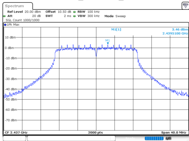
802.11n20_2437MHz_Chain 0
