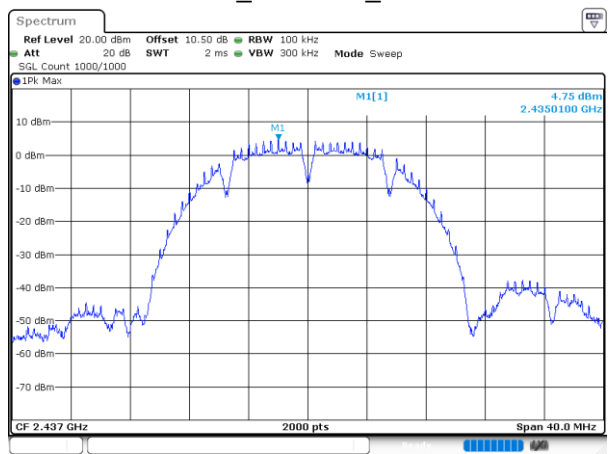
802.11b_2437MHz_Chain 1
