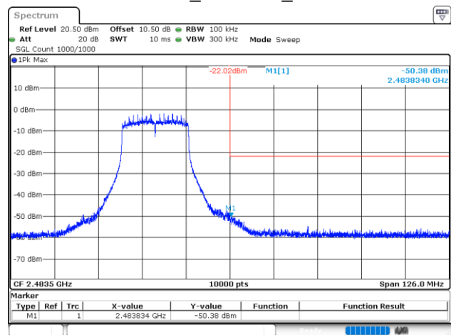
802.11n20_2462MHz_Chain 1
