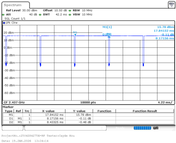
802.11b_2437MHz_Chain 1
