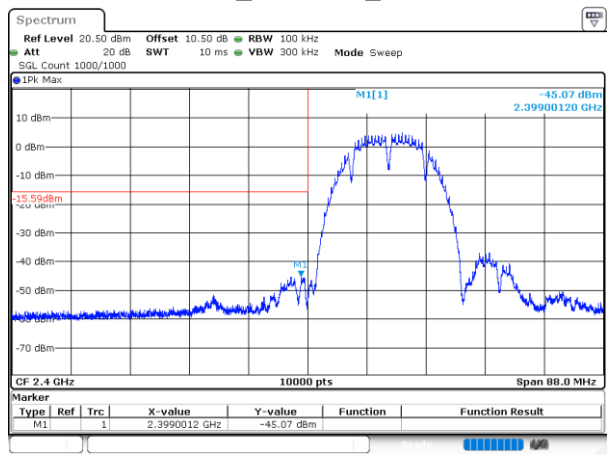
802.11b_2412MHz_Chain 1
