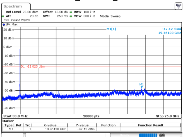
802.11n20_2462MHz_Chain 1
