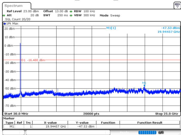
802.11n20_2412MHz_Chain 0
