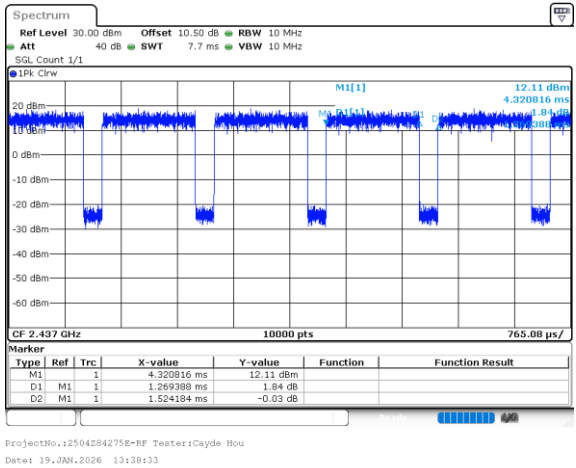
802.11n20_2437MHz_Chain 1
