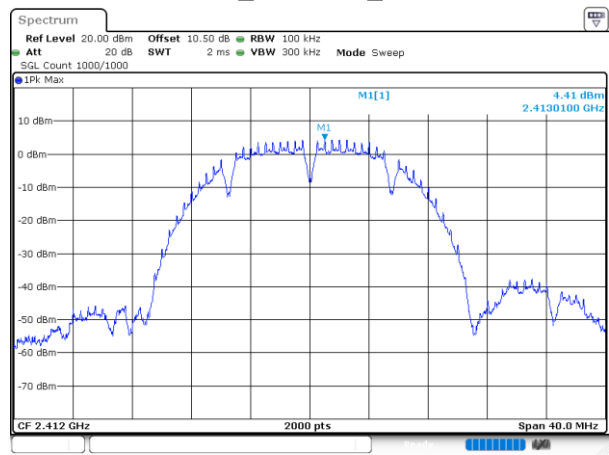
802.11b_2412MHz_Chain 1
