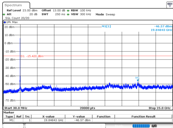
802.11b_2462MHz_Chain 1
