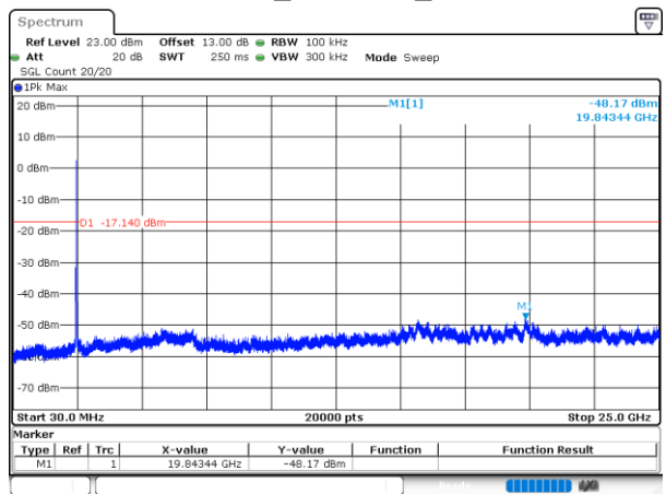
802.11n20_2462MHz_Chain 0
