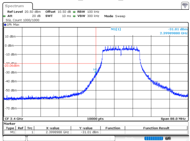
802.11n20_2412MHz_Chain 1
