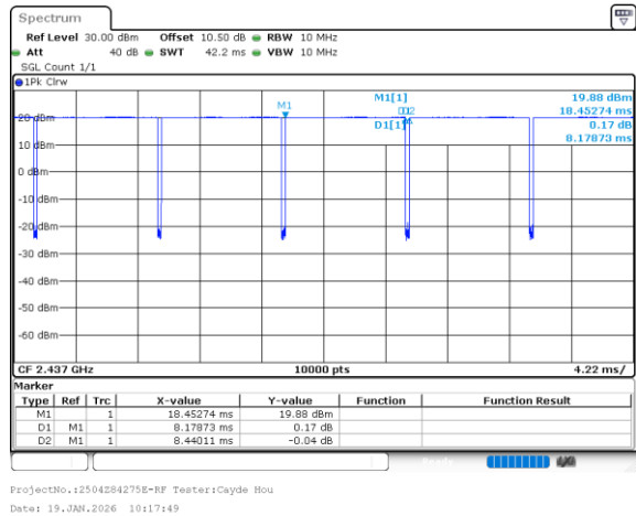
802.11b_2437MHz_Chain 0
