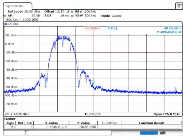
802.11b_2462MHz_Chain 0
