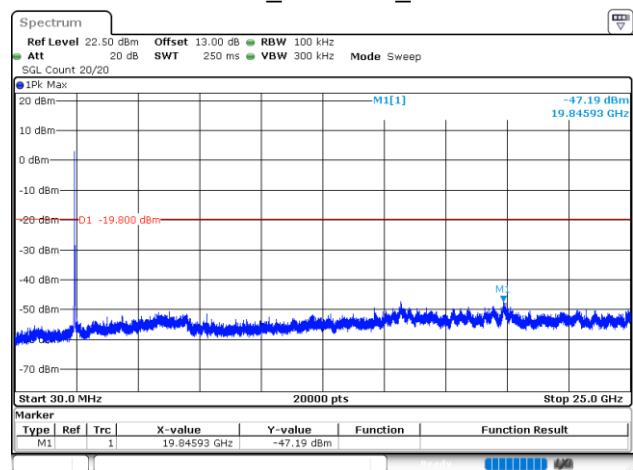
802.11n20_2437MHz_Chain 1
