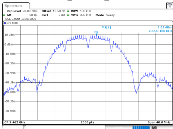
802.11b_2462MHz_Chain 0
