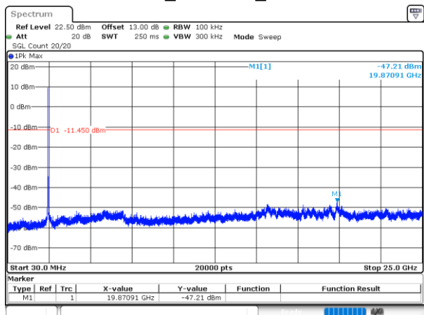
802.11b_2437MHz_Chain 0
