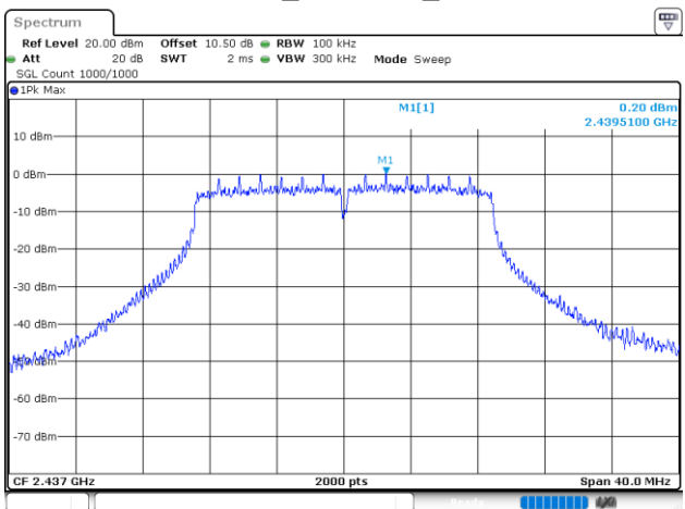
802.11n20_2437MHz_Chain 1
