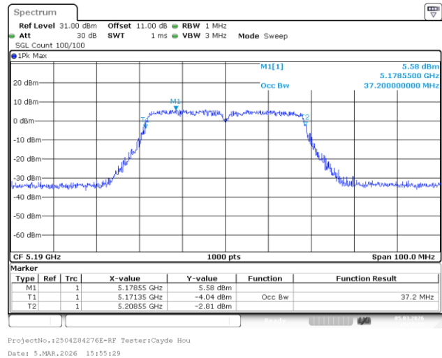
802.11ac40_5190MHz_Chain 1
