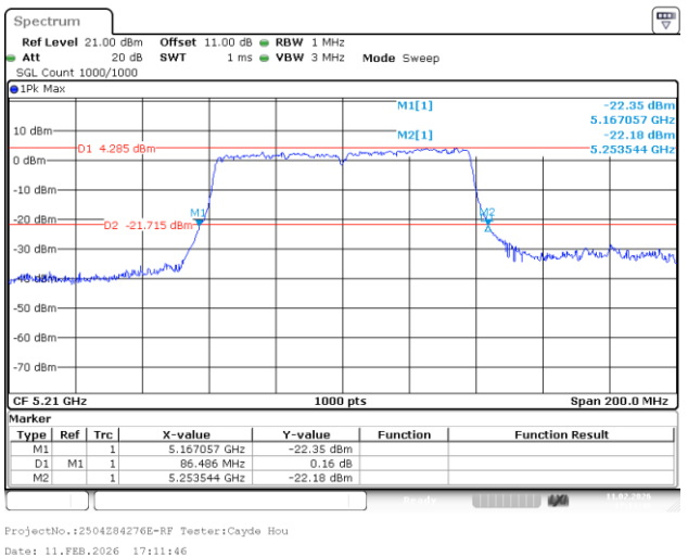
802.11ac80_5210MHz_Chain 1
