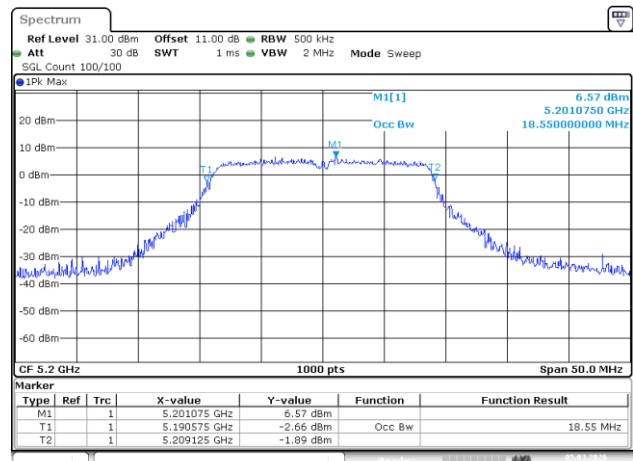
802.11ac20_5200MHz_Chain 1
