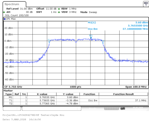
802.11ac40_5755MHz_Chain 1
