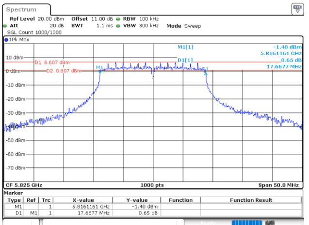
802.11ac20_5825MHz_Chain 1
