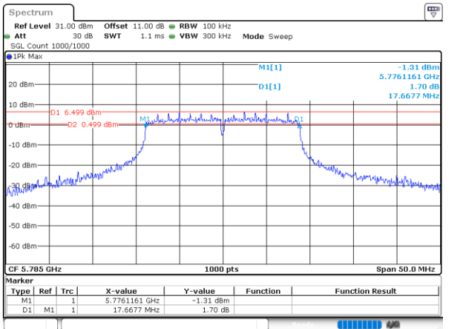
802.11ac20_5785MHz_Chain 0
