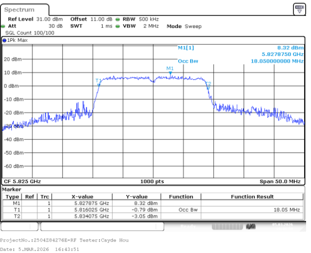
802.11ac20_5825MHz_Chain 1
