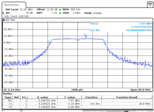
802.11ac20_5240MHz_Chain 1
