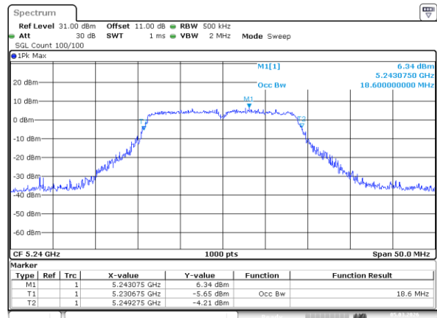
802.11ac20_5240MHz_Chain 0
