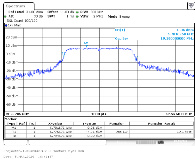
802.11ac20_5785MHz_Chain 1
