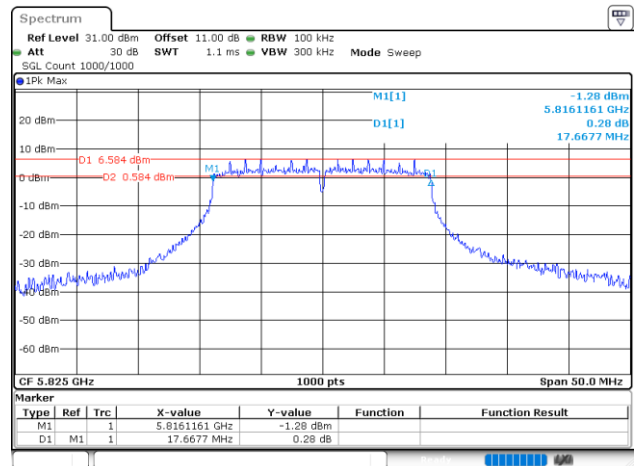
802.11ac20_5825MHz_Chain 0
