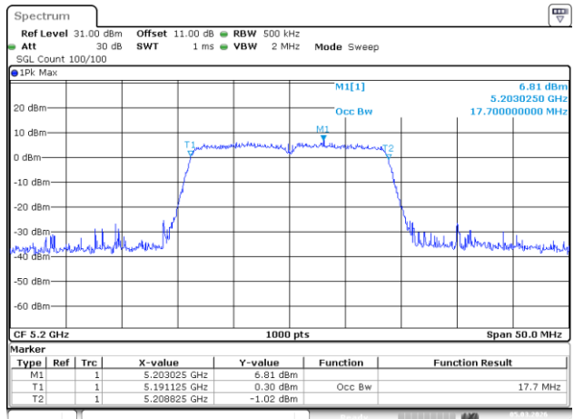
802.11ac20_5200MHz_Chain 0
