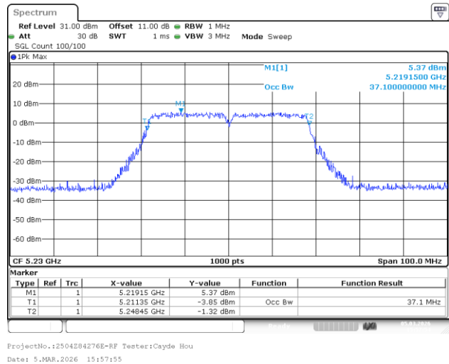
802.11ac40_5230MHz_Chain 1
