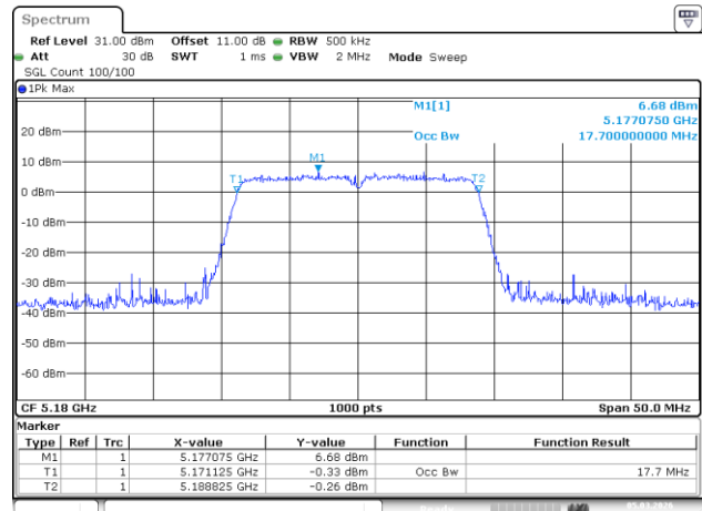
802.11ac20_5180MHz_Chain 0
