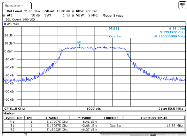
802.11ac20_5180MHz_Chain 1
