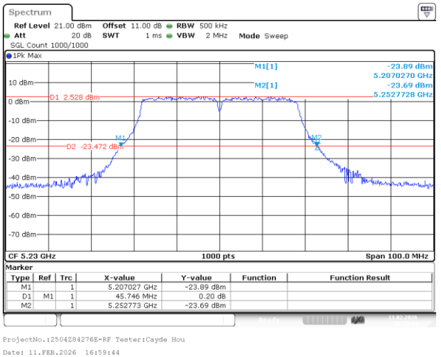
802.11ac40_5230MHz_Chain 1
