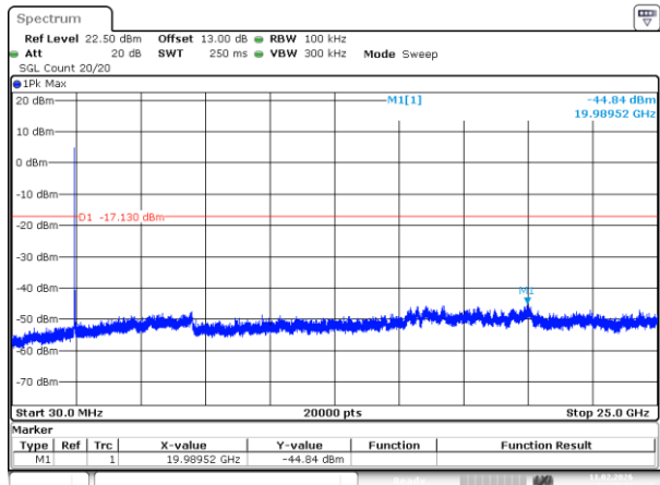
802.11b_2437MHz_Chain 0
