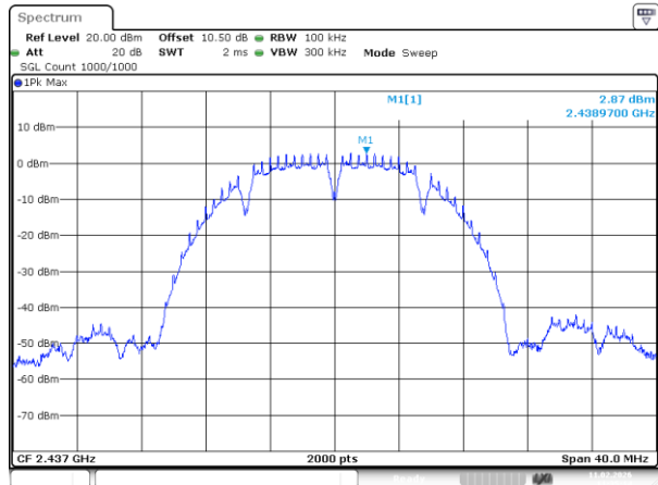
802.11b_2437MHz_Chain 0
