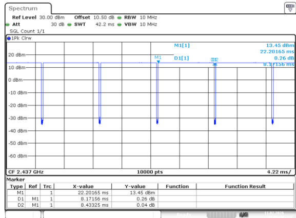
802.11b_2437MHz_Chain 0
