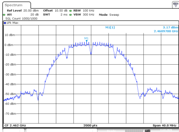
802.11b_2462MHz_Chain 0
