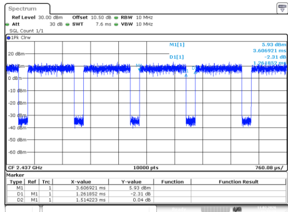
802.11n20_2437MHz_Chain 0
