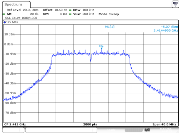
802.11n20_2412MHz_Chain 1
