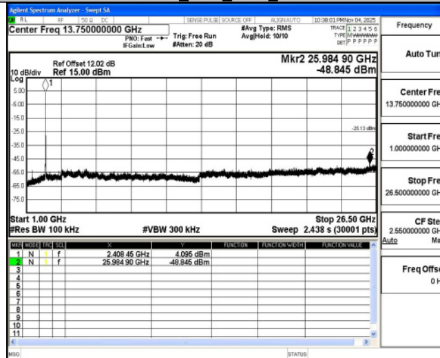
11N20MIMO_Ant2_2412_0~Reference
