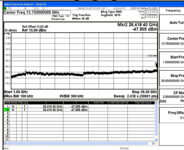
11N40MIMO_Ant2_2437_0~Reference
