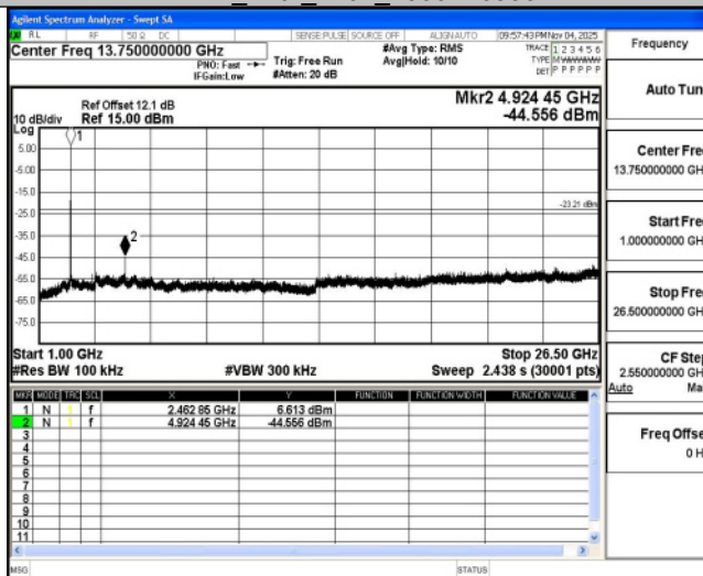
11B_Ant2_2462_0~Reference
