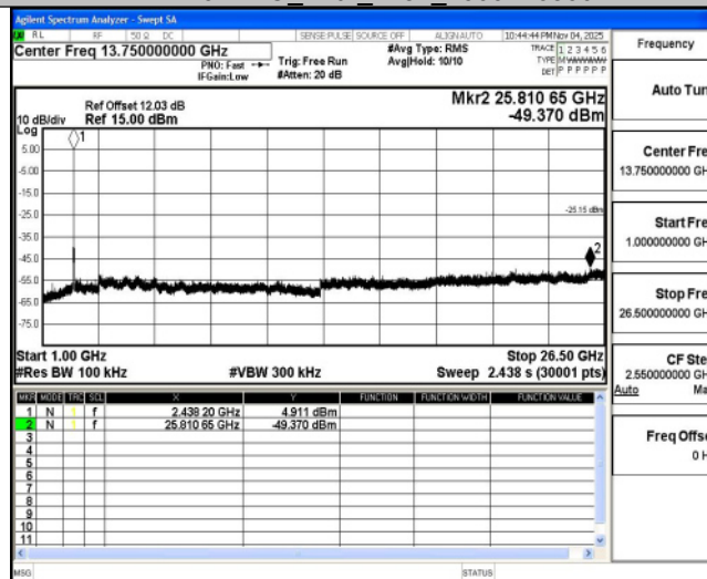
11N20MIMO_Ant2_2437_0~Reference
