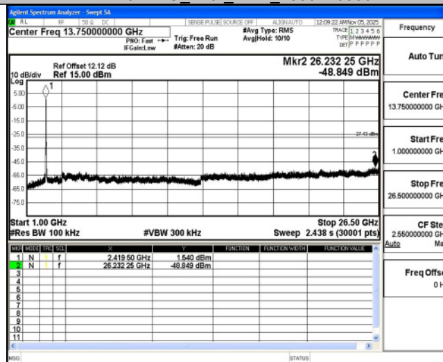
11N40MIMO_Ant1_2437_0~Reference
