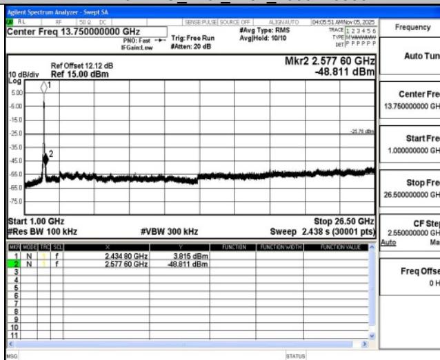
11N40MIMO_Ant1_2452_0~Reference
