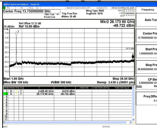
11AX40MIMO_Ant1_2437_0~Reference
