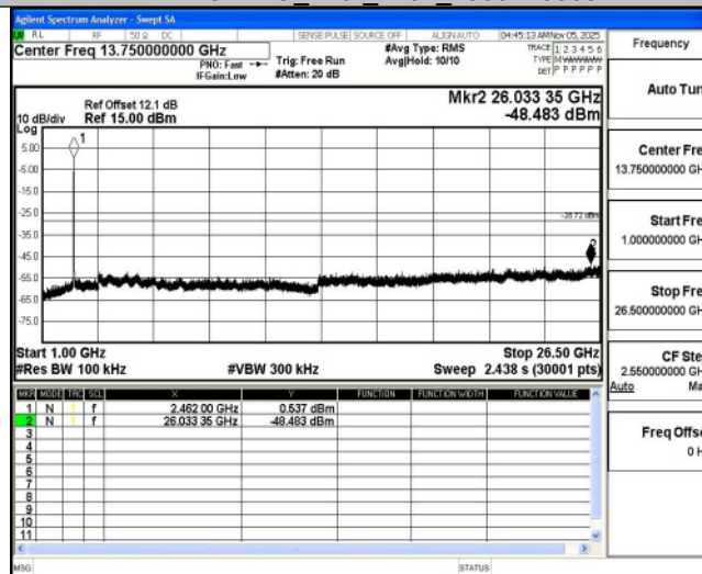
11AX20MIMO_Ant2_2462_0~Reference
