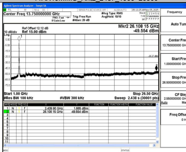
11AX40MIMO_Ant1_2452_0~Reference
