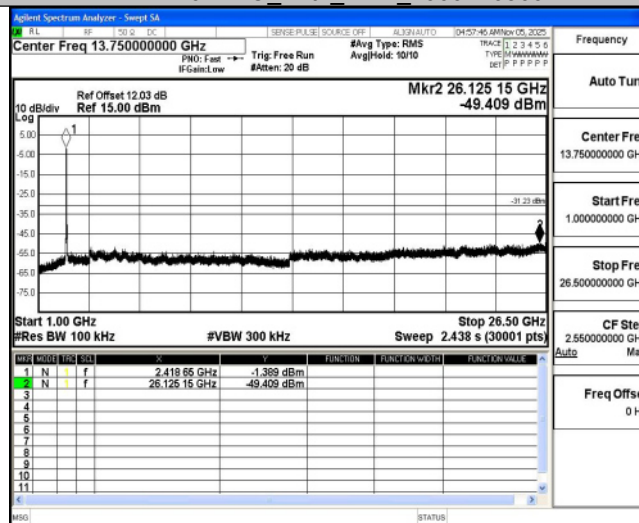
11AX40MIMO_Ant2_2422_0~Reference
