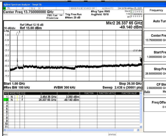
11N40MIMO_Ant2_2452_0~Reference
