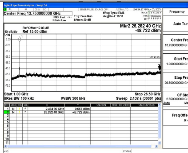
11AX20MIMO_Ant2_2437_0~Reference
