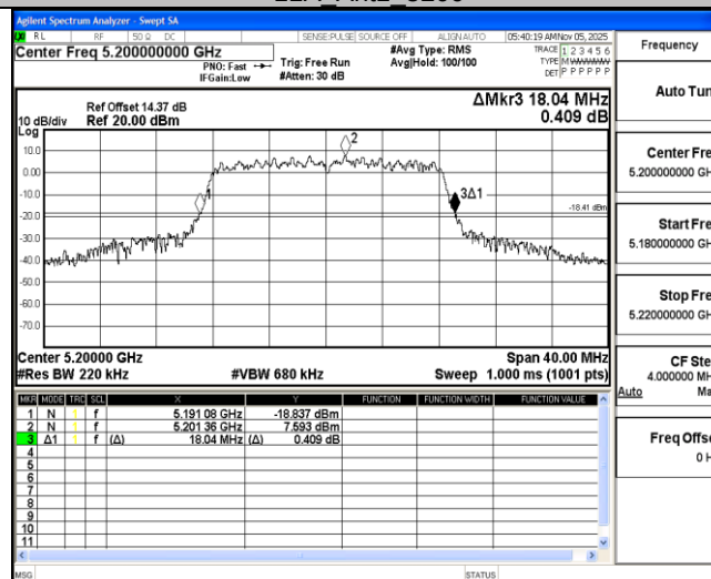
11A_Ant2_5200
