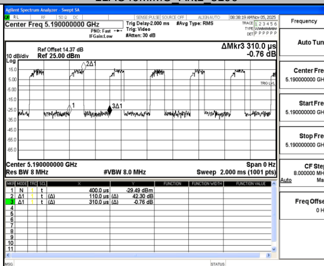
11AC40MIMO_Ant2_5190
