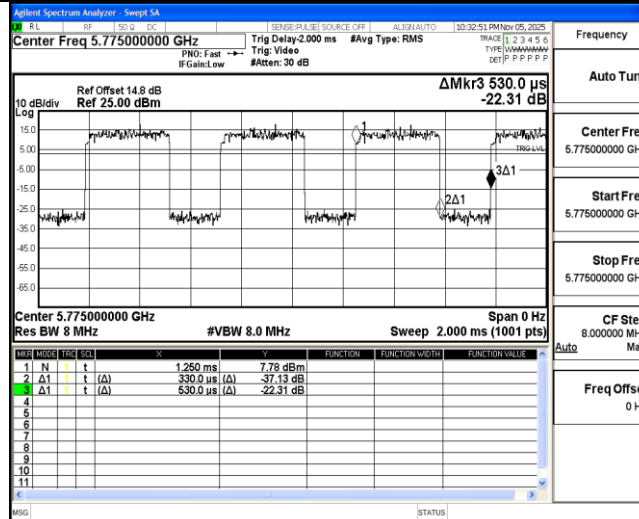
11AX80MIMO_Ant2_5775
