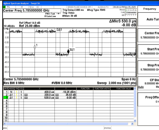
11AX20MIMO_Ant2_5785
