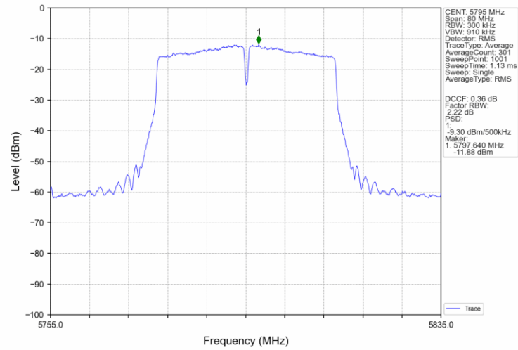
802.11n(HT40)_HCH_5795MHz_MIMO_NTNV
