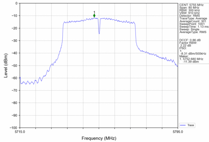
802.11ac(VHT40)_LCH_5755MHz_MIMO_NTNV
