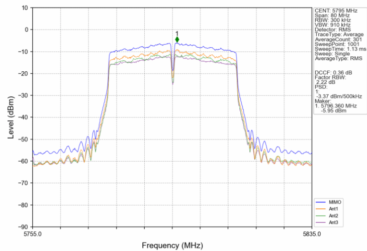
802.11n(HT40)_HCH_5795MHz_MIMO_NTNV
