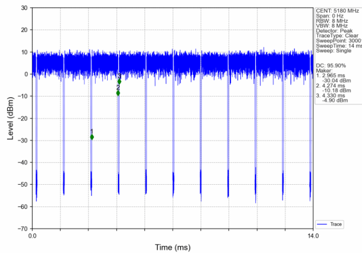
802.11n(HT20) LCH 5180MHz_NTNV
