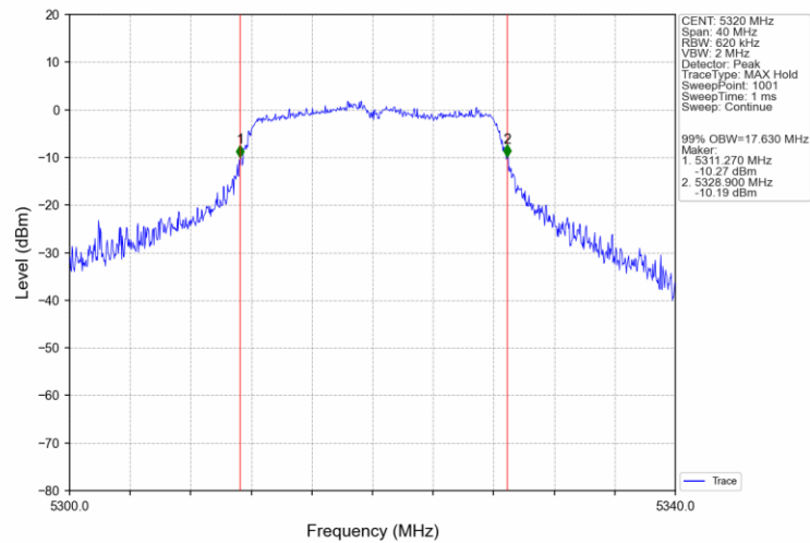
802.11a_HCH_5320MHz_Ant2_NTNV
