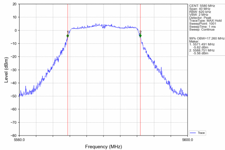
802.11a_MCH_5580MHz_Ant2_NTNV
