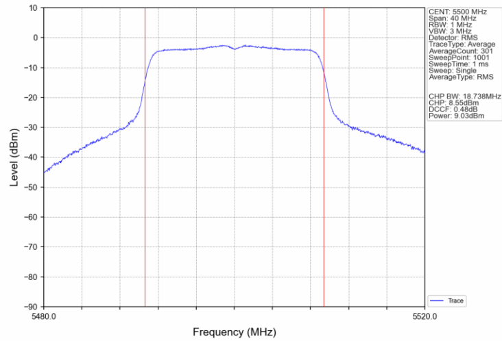
802.11ac(VHT20)_LCH_5500MHz_Ant4_NTNV
