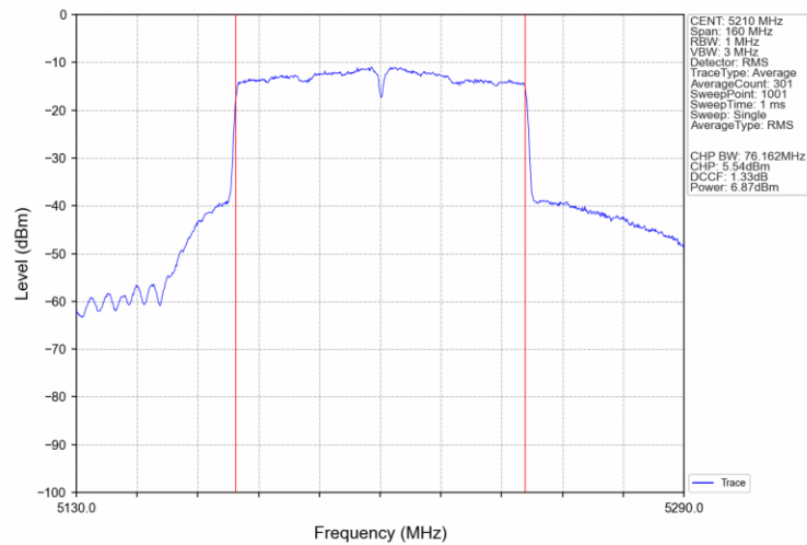
802.11ac(VHT80)_MCH_5210MHz_Ant4_NTNV
