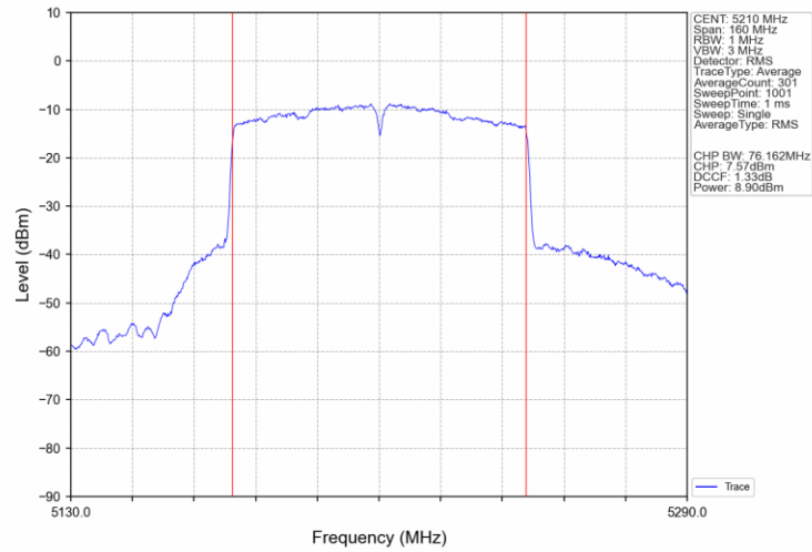
802.11ac(VHT80)_MCH_5210MHz_Ant4_NTNV
