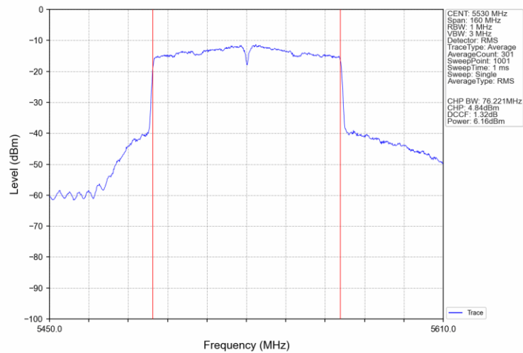
802.11ac(VHT80)_LCH_5530MHz_Ant4_NTNV
