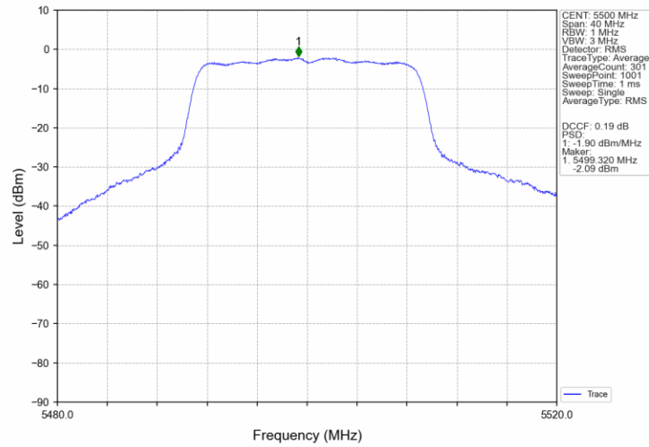
802.11n(HT20)_LCH_5500MHz_Ant3_NTNV
