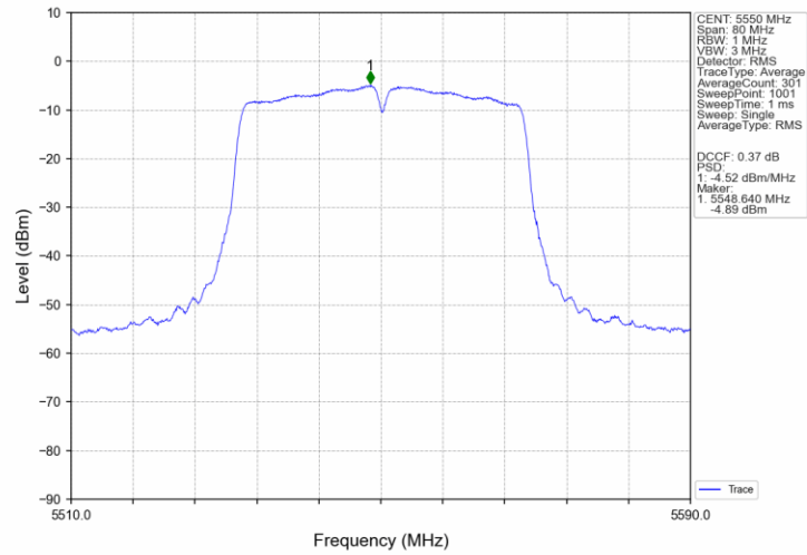
802.11n(HT40)_MCH_5550MHz_MIMO_NTNV
