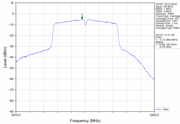
802.11n(HT40)_HCH_5310MHz MIMO NTN
