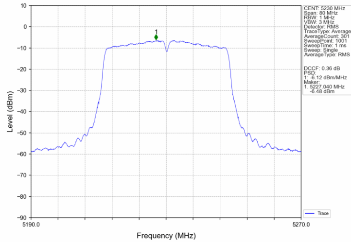
802.11n(HT40)_HCH_5230MHz_Ant3_NTNV
