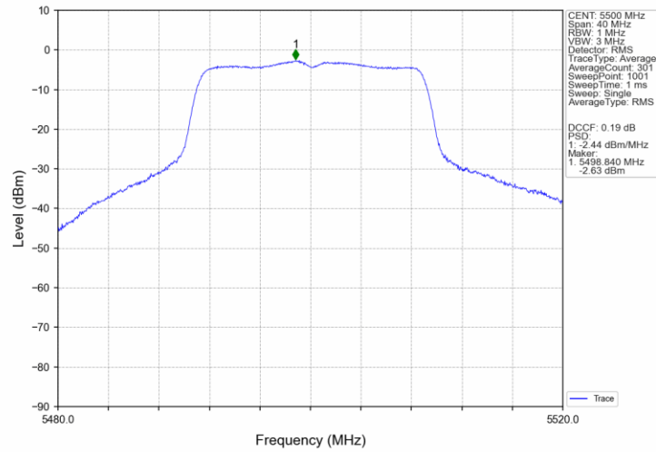
802.11n(HT20)_LCH_5500MHz_MIMO_NTNV
