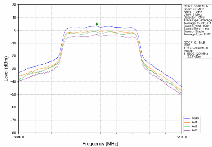
802.11n(HT20)_HCH_5700MHz MIMO NTN
