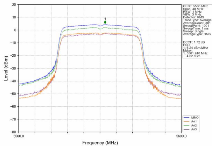
802.11ax(HEW20) MCH 5580MHz SU / MIMO NTN
