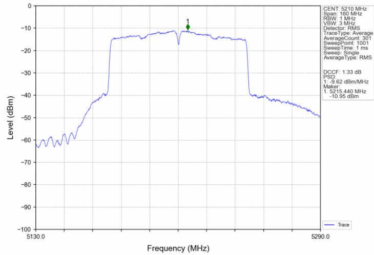
802.11ac(VHT80)_MCH_5210MHz_Ant3_NTNV
