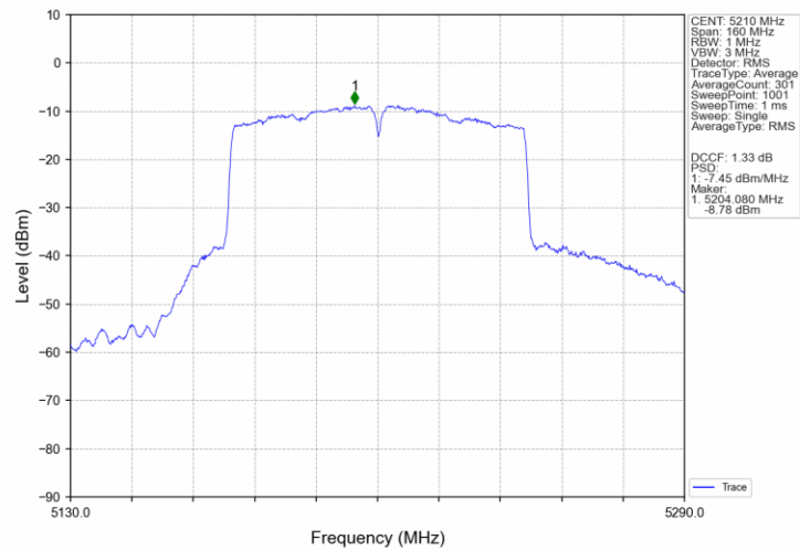
802.11ac(VHT80)_MCH_5210MHz_Ant3_NTNV
