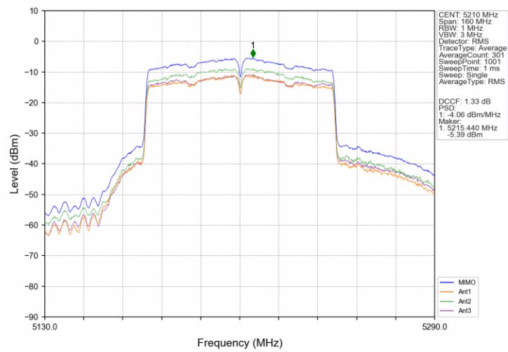
802.11ac(VHT80)_MCH_5210MHz_MIMO_NTNV
