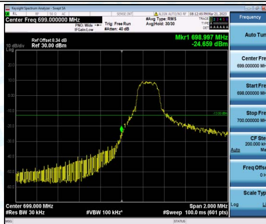
Band12-1.4MHz-16QAM-23017-1-0-Low--24.66-PASS
