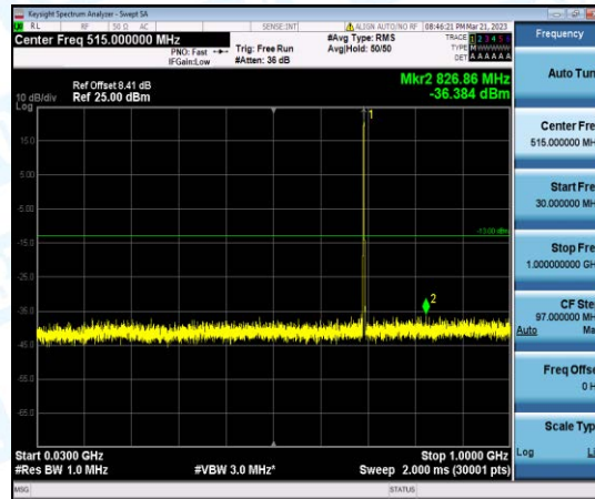
Band12-3MHz-QPSK-23025-1-0-Low-30-1000--36.38-PASS
