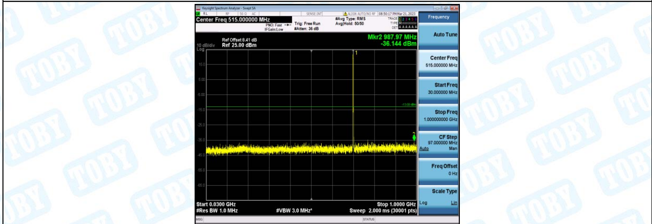
Band12-3MHz-QPSK-23095-1-0-Low-30-1000--36.14-PASS
