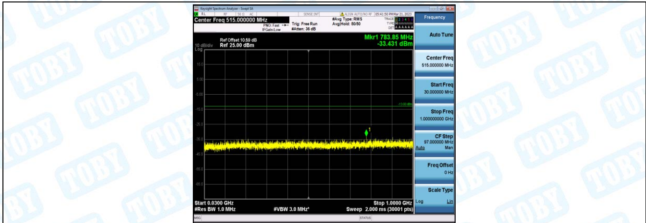
Band2-20MHz-QPSK-18700-1-0-Low-30-1000--33.43-PASS
