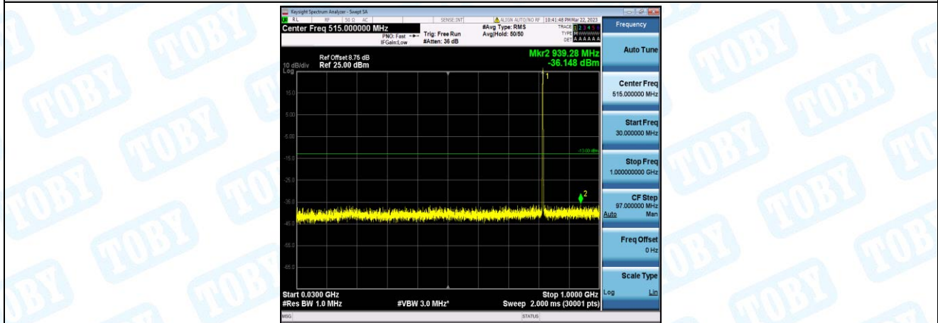
Band26-3MHz-16QAM-26740-1-0-Low-30-1000--36.15-PASS
