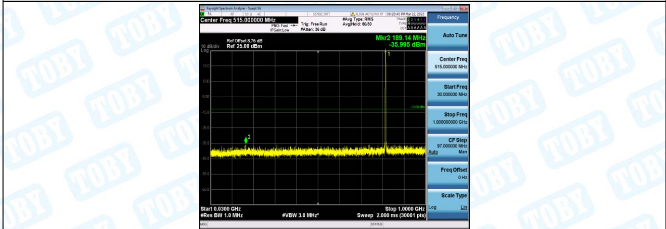
Band26-1.4MHz-QPSK-26740-1-0-Low-30-1000--36-PASS
