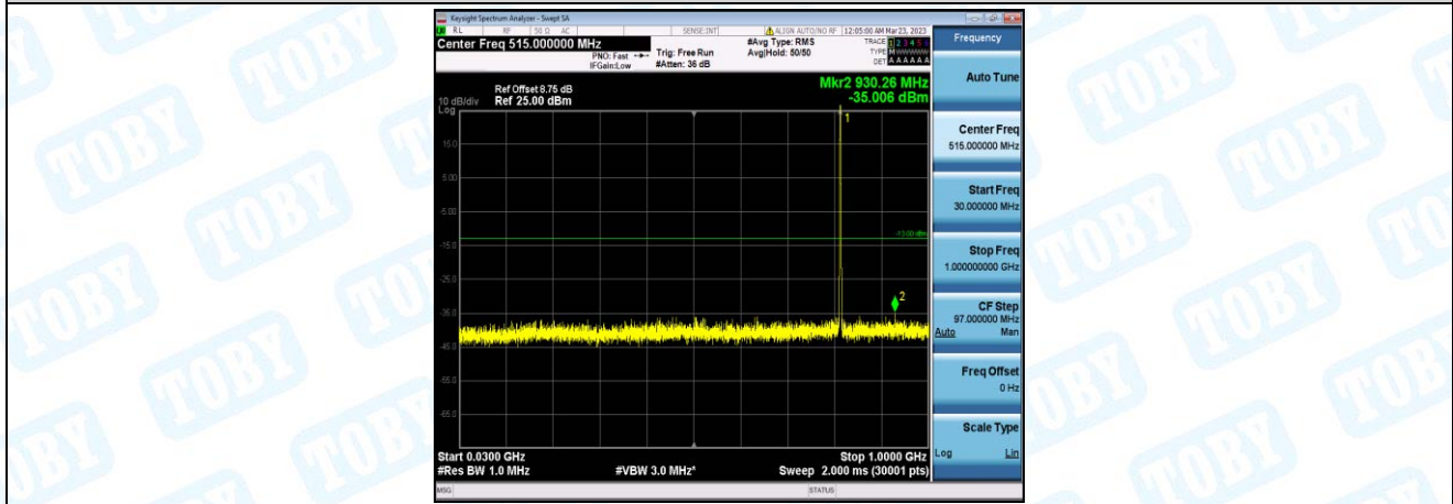
Band26-5MHz-QPSK-26740-1-0-Low-30-1000--35.01-PASS
