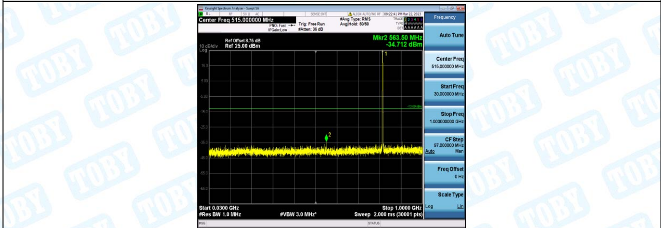
Band26-1.4MHz-16QAM-26740-1-0-Low-30-1000--34.71-PASS
