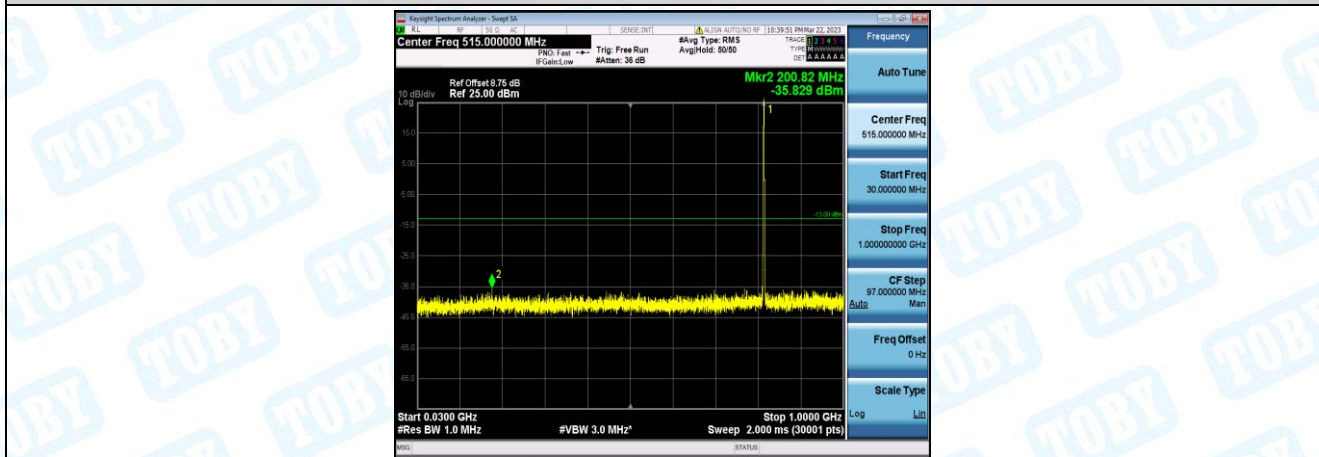
Band26-3MHz-QPSK-26740-1-0-Low-30-1000--35.83-PASS
