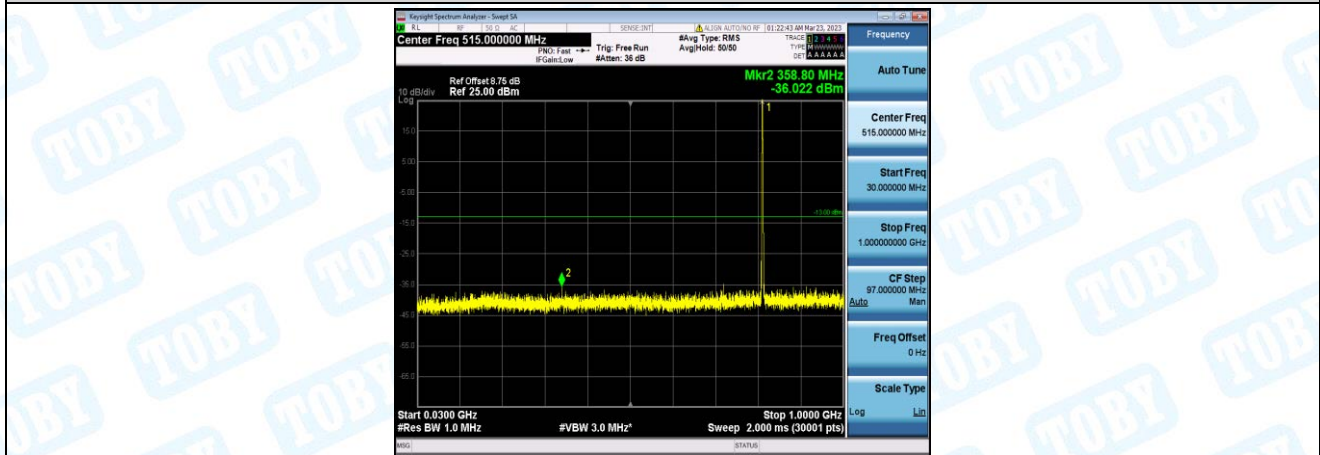
Band26-10MHz-16QAM-26740-1-0-Low-30-1000--36.02-PASS
