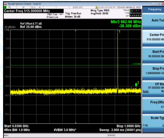
Band26-10MHz-QPSK-26840-1-0-Low-30-1000--36.31-PASS
