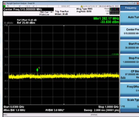
Band4-20MHz-QPSK-20050-1-0-Low-30-1000--33.83-PASS
