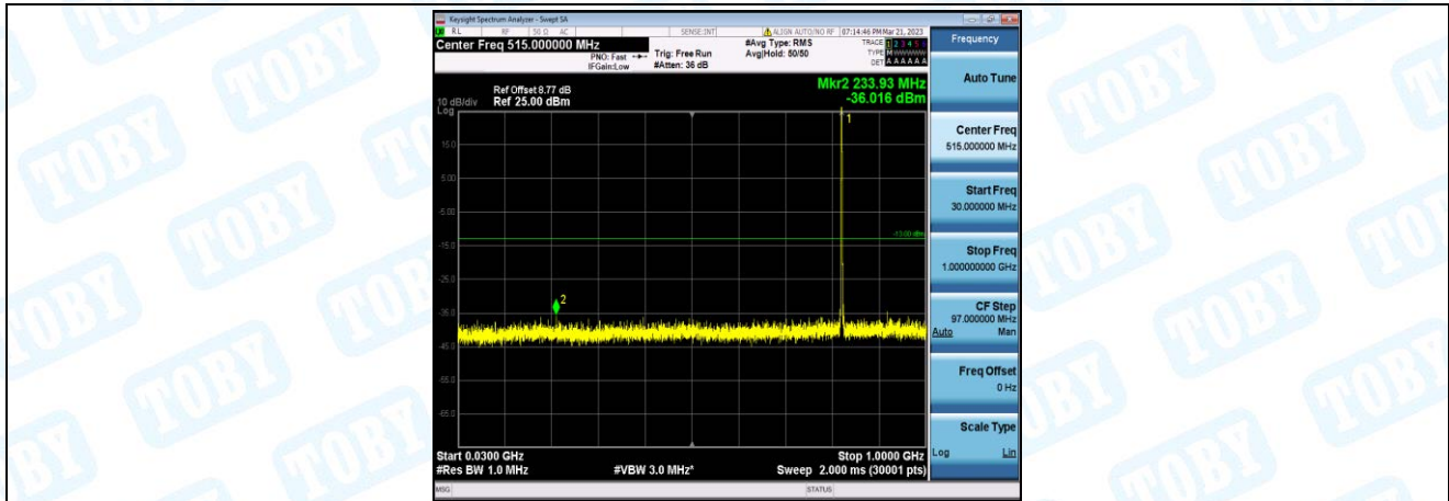
Band5-5MHz-QPSK-20425-1-0-Low-30-1000--36.02-PASS
