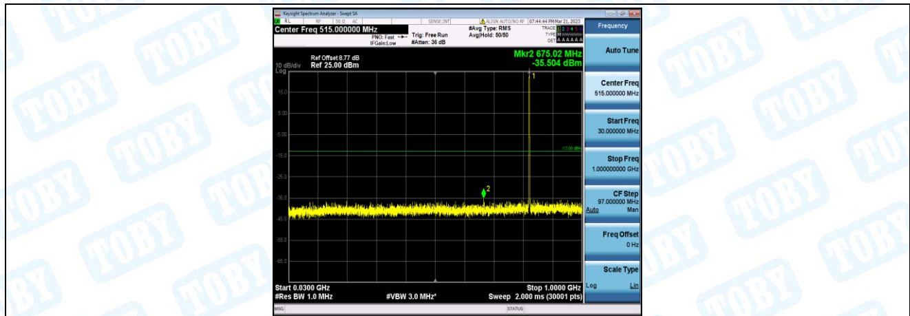
Band5-10MHz-QPSK-20450-1-0-Low-30-1000--35.5-PASS
