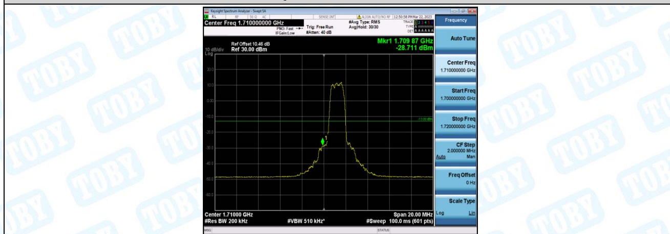
Band66-10MHz-QPSK-132022-6-0-Low--28.71-PASS
