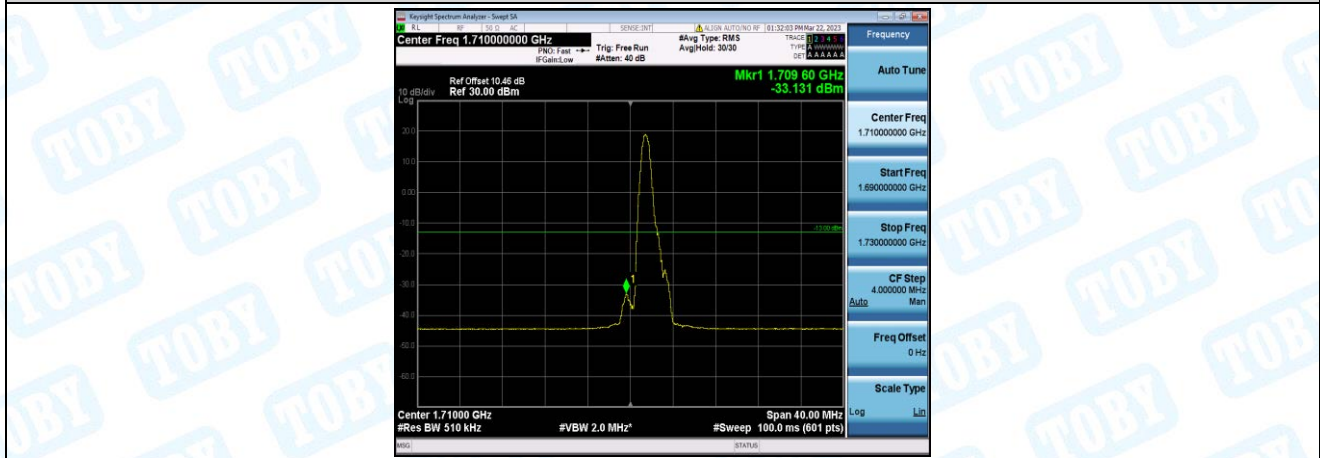
Band66-20MHz-QPSK-132072-1-0-Low--33.13-PASS
