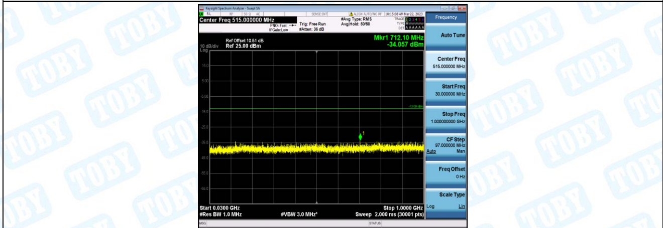
Band66-3MHz-QPSK-132322-1-0-Low-30-1000--34.06-PASS
