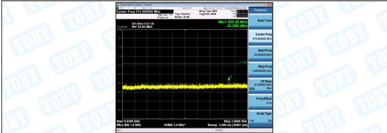
Band66-10MHz-QPSK-132322-1-0-Low-30-1000--33.01-PASS
