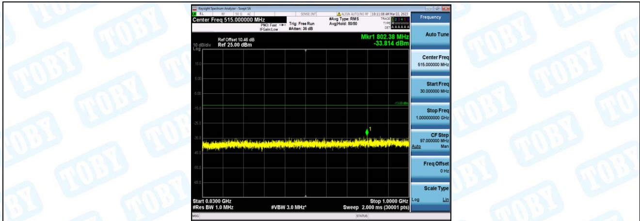
Band66-3MHz-QPSK-131987-1-0-Low-30-1000--33.81-PASS
