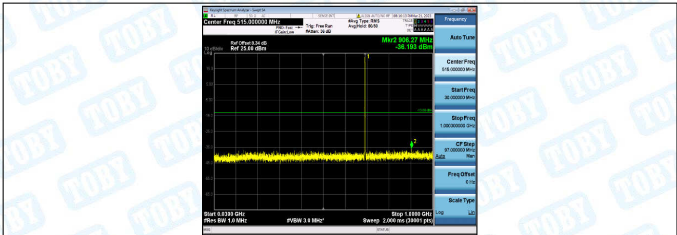
Band12-1.4MHz-16QAM-23017-1-0-Low-30-1000--36.19-PASS
