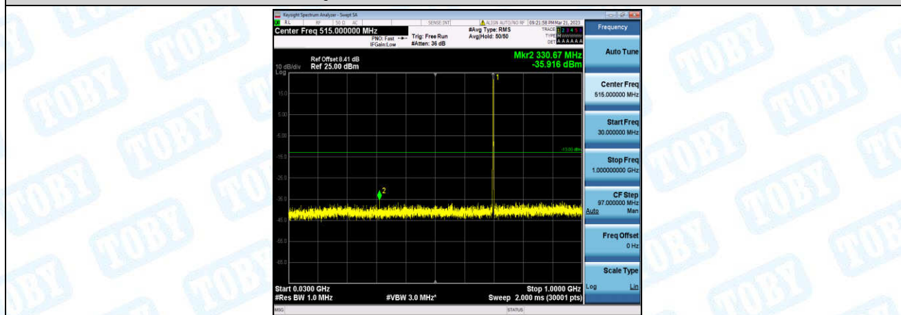
Band12-5MHz-QPSK-23095-1-0-Low-30-1000--35.92-PASS
