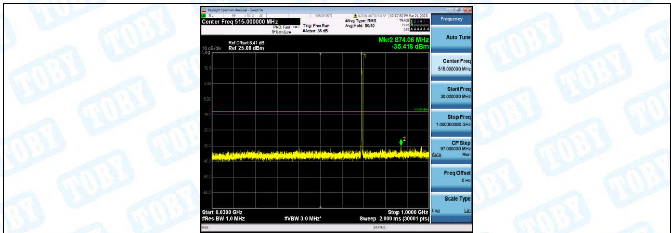
Band12-10MHz-QPSK-23060-1-0-Low-30-1000--35.42-PASS
