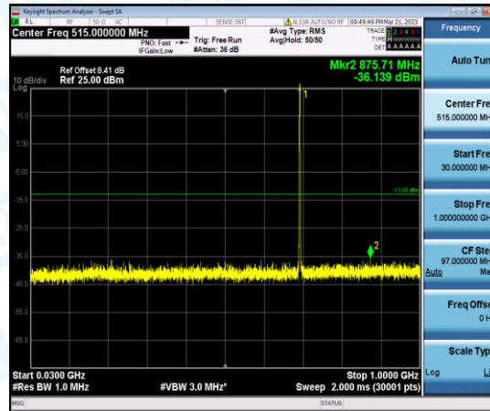
Band12-10MHz-16QAM-23060-1-0-Low-30-1000--36.14-PASS
