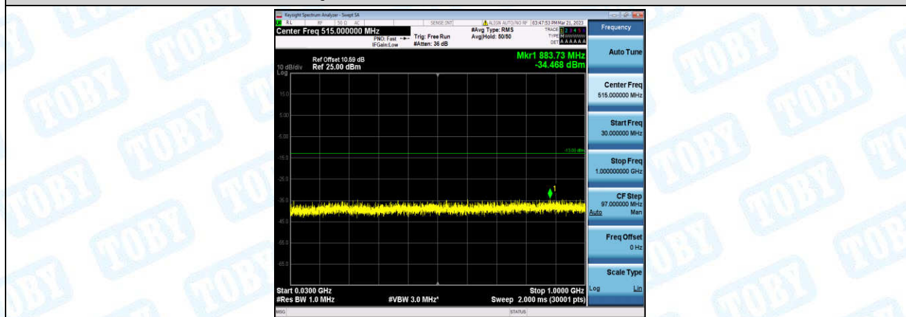
Band2-3MHz-QPSK-18900-1-0-Low-30-1000--34.47-PASS
