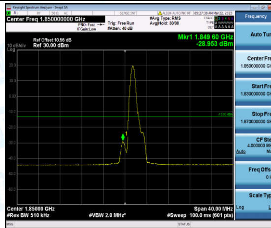
Band25-20MHz-QPSK-26140-1-0-Low--28.95-PASS
