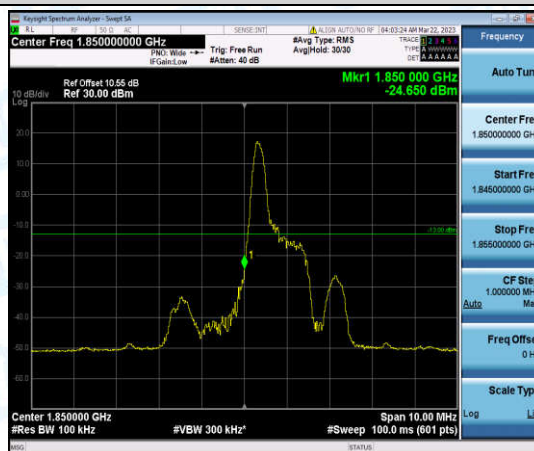
Band25-5MHz-QPSK-26065-1-0-Low--24.65-PASS
