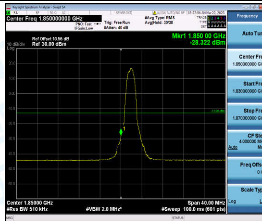
Band25-20MHz-QPSK-26140-6-0-Low--28.32-PASS
