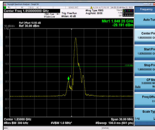
Band25-15MHz-QPSK-26115-1-0-Low--29.19-PASS
