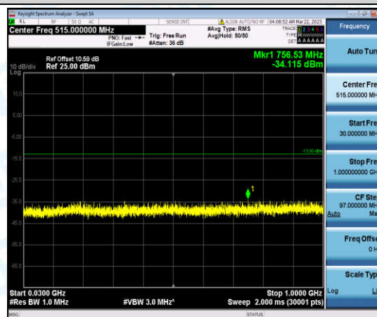
Band25-5MHz-QPSK-26365-1-0-Low-30-1000--34.12-PASS
