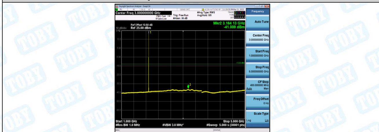
Band25-1.4MHz-QPSK-26365-1-0-Low-1000-5000--41.01-PASS
