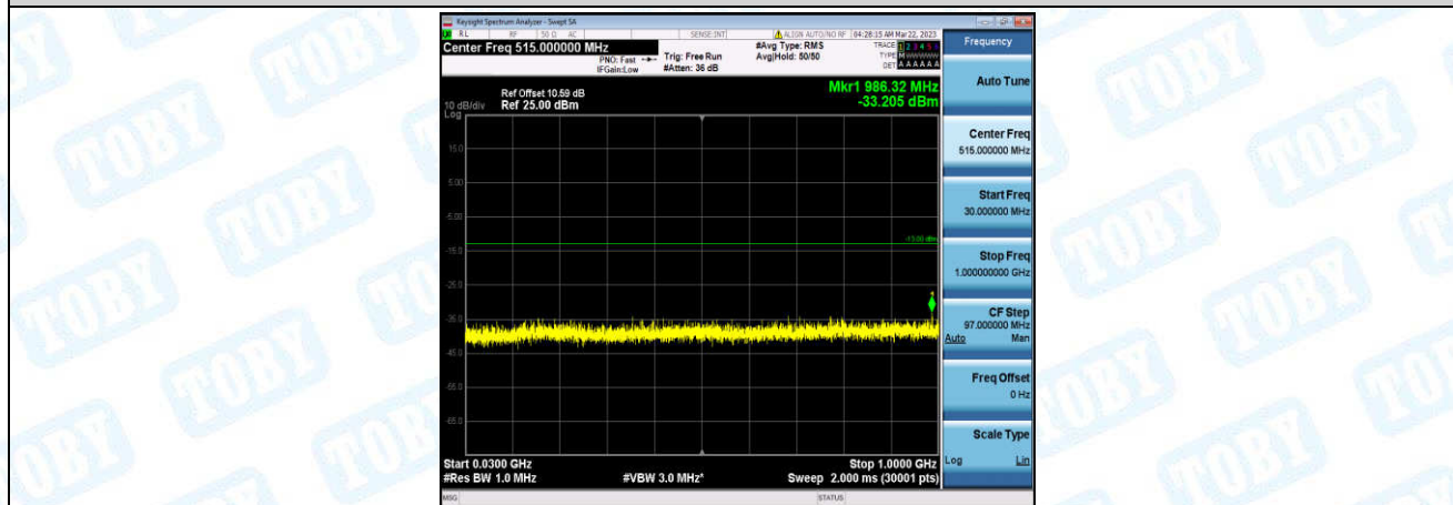
Band25-10MHz-QPSK-26365-1-0-Low-30-1000--33.21-PASS
