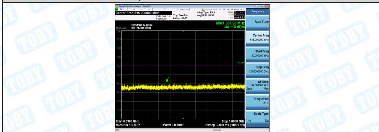
Band25-15MHz-QPSK-26365-1-0-Low-30-1000--34.11-PASS
