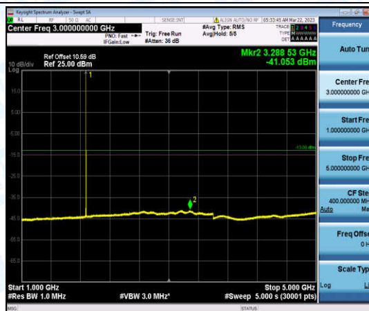
Band25-20MHz-QPSK-26365-1-0-Low-1000-5000--41.05-PASS
