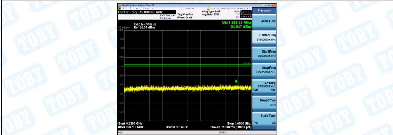
Band25-20MHz-16QAM-26365-1-0-Low-30-1000--34.05-PASS
