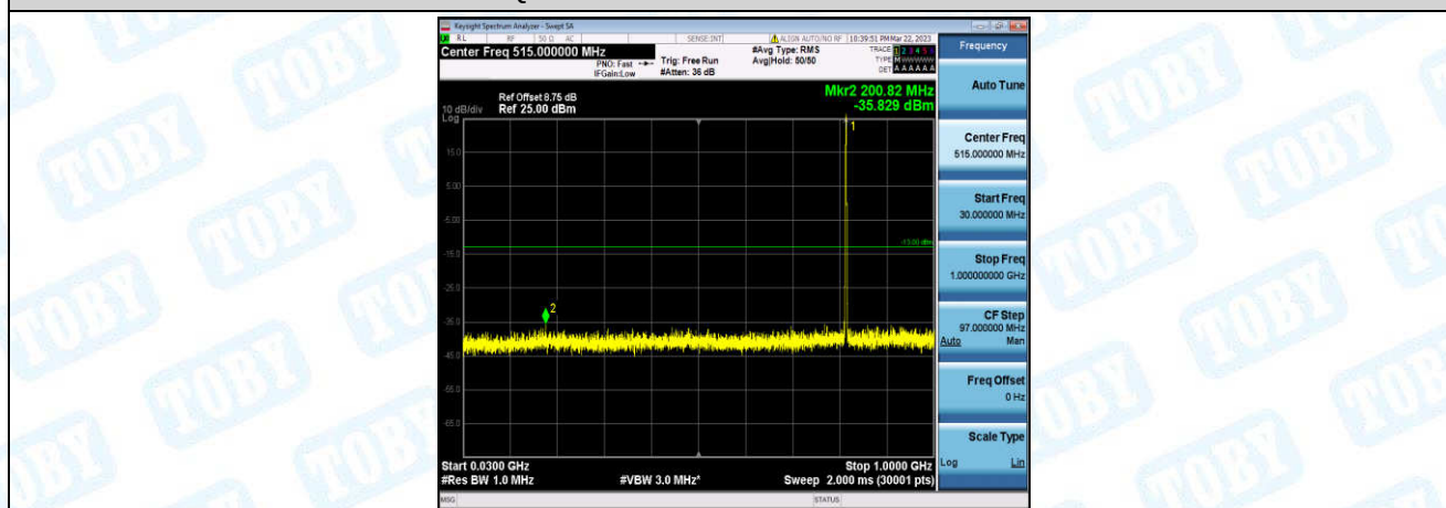
Band26-3MHz-QPSK-26740-1-0-Low-30-1000--35.83-PASS
