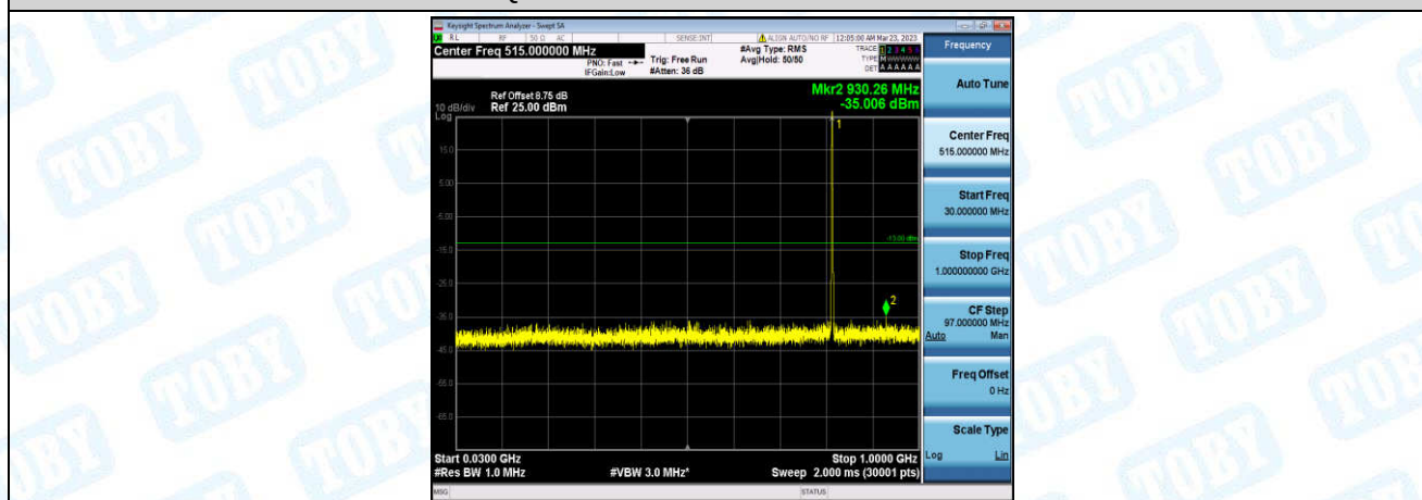
Band26-5MHz-QPSK-26740-1-0-Low-30-1000--35.01-PASS
