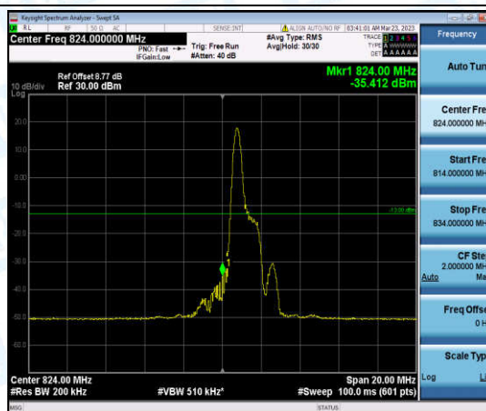
Band26-10MHz-QPSK-26840-1-0-Low--35.41-PASS
