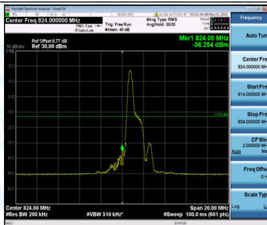
Band26-10MHz-16QAM-26840-1-0-Low--36.25-PASS
