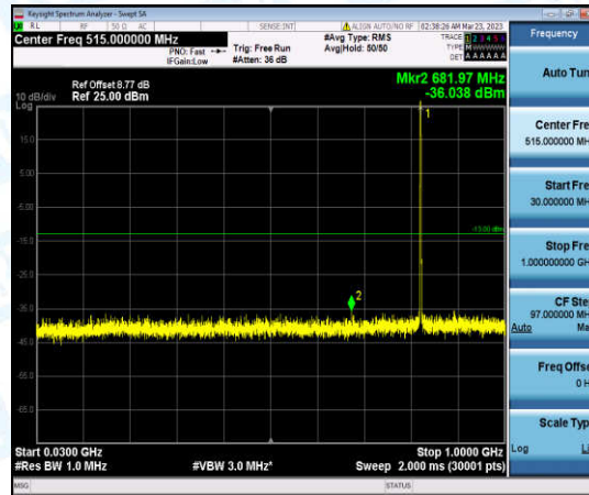
Band26-3MHz-QPSK-26805-1-0-Low-30-1000--36.04-PASS
