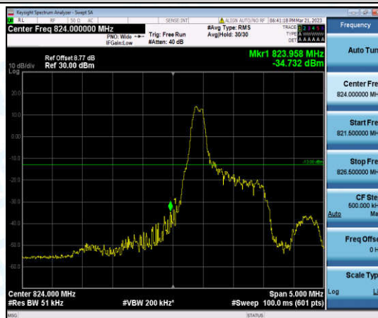
Band5-3MHz-QPSK-20415-1-0-Low--34.73-PASS
