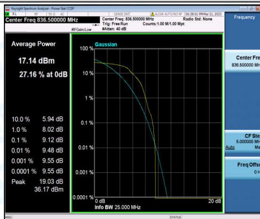
Band5-3MHz-QPSK-20525-1-0-Low-9.12-≤13-PASS
